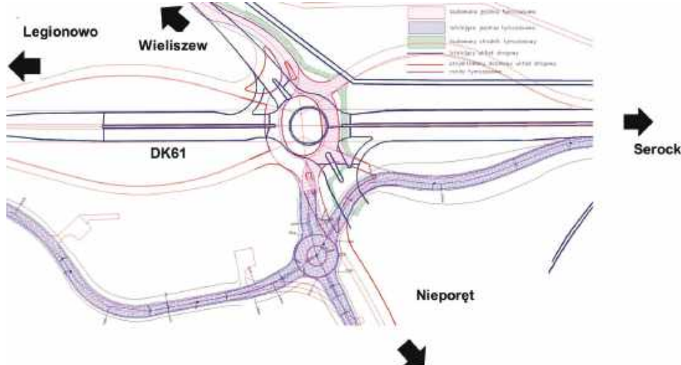
Schemat ronda tymczasowego na DK61
