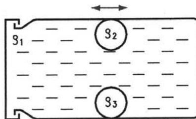
Rys. 5. Prosty przyrząd do pokazu pływania kulek w układzie poruszającym się ruchem przyspieszonym, \rho_1 – gęstość cieczy wypełniającej słojek, \rho_2, \rho_3 – gęstości zanurzonych w niej kulek.
