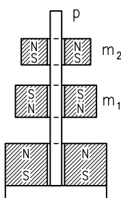
Rys. 10. Układ do badania zderzenia kulek o masach m_1 , m_2 , prowadzonych wzdłuż pionowego pręta p, pokazany w przekroju osiowym.
