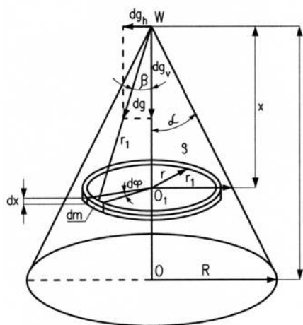
Rys. 3. Stożek wraz z elementarnym pierścieniem, wyodrębnionym w celu obliczenia natężenia pola grawitacyjnego; dg – elementarny przyczynnik do natężenia pola grawitacyjnego od elementu masy dm , dg_v , dg_h – składowe przyczynki dg odpowiednio: pionowa i pozioma, \rho – gęstość materiału stożka.
