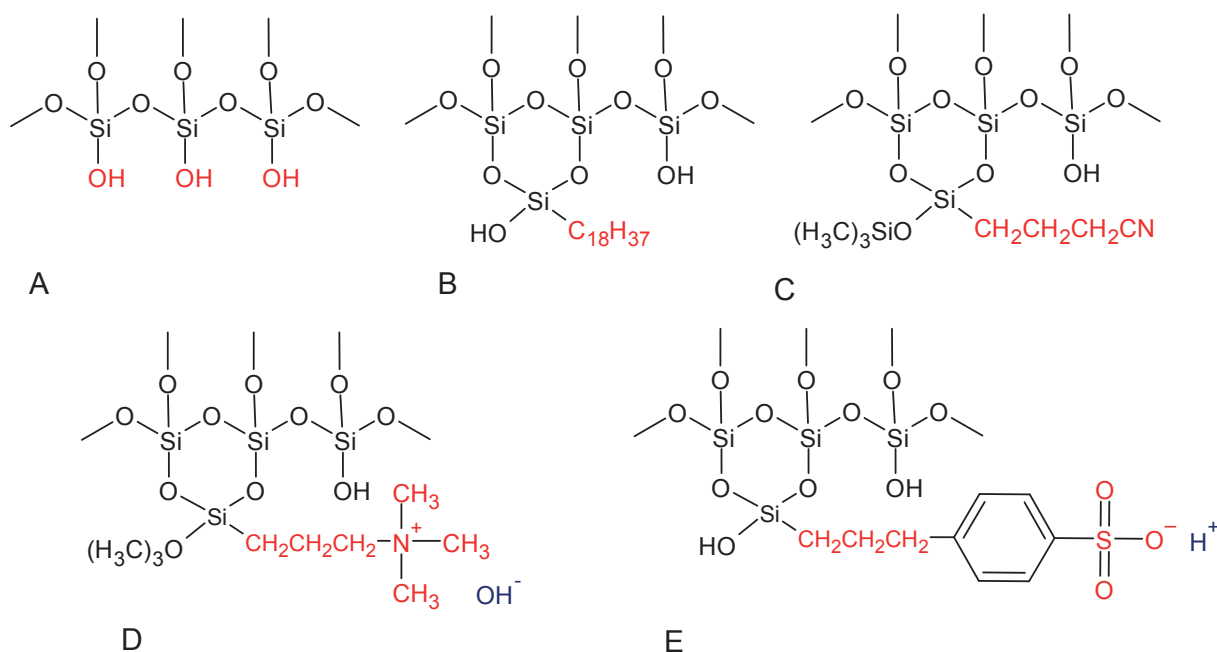
Rysunek 3. Fragment struktury żelu krzemionkowego z zaznaczonymi: na czerwono – centrami aktywnymi, na niebiesko – przeciwnymi; A – niemodyfikowany żel krzemionkowy o właściwościach polarnych, B – żel krzemionkowy nasycony długimi łańcuchami węglowodorowymi o niepolarnym charakterze, C – żel krzemionkowy modyfikowany grupami cyjanopropylowymi o porównywalnym powinowactwie do substancji polarnych i niepolarnych, D – żel krzemionkowy związany z anionitem (np. N, N, N -trimetylo, N -propyloamina), E – żel krzemionkowy związany z kationitem (np. kwas 4 – propylsulfonowy).
