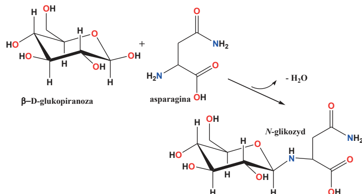
Rysunek 8. Schemat reakcji Maillarda
