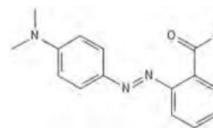
Rys. 2 – Wzór strukturalny czerwieni metylowej
