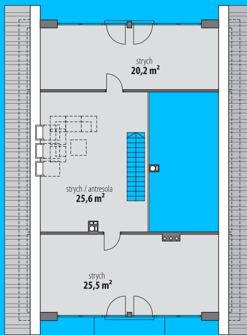
Poddasze
