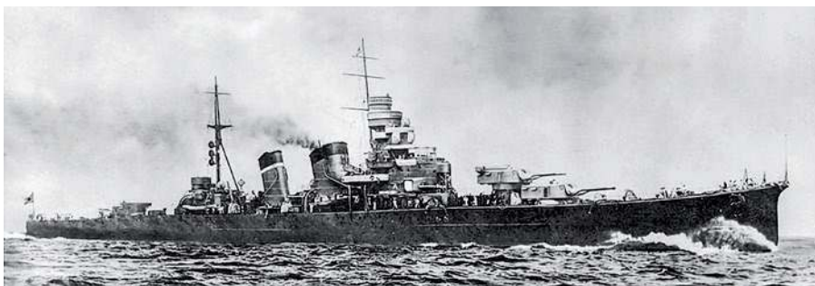
▲ Aoba w początkowym okresie służby w oryginalnej konfiguracji. Wyraźnie widoczne podobieństwo w kształcie kadłuba i głównej nadbudówki do typu Furutaka .
