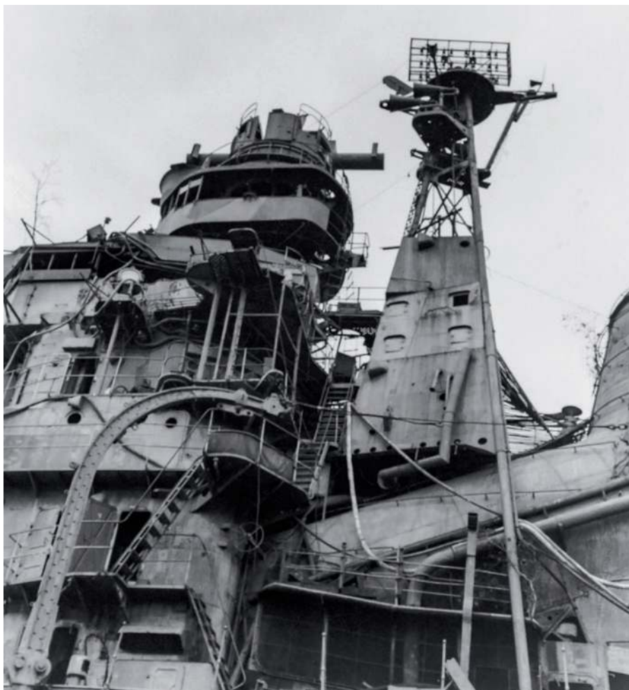
▲ Widok na główną nadbudówkę i przedni maszt Aoby . Na szczycie nadbudówki widoczna jest wieżyczka z dalmierzem oraz director dla artylerii głównej. Trójnożny maszt przedni zainstalowano w miejsce oryginalnego podczas naprawy po bitwie koło przylądka Esperance. Na jego szczycie znajduje się antena radaru dozoru powietrznego Typ 21. Zdjęcie wykonane po wojnie, w październiku 1945 r., gdy wrak Aoby znajdował się w Kure.
