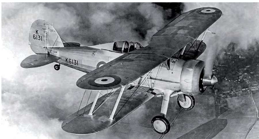
▲ Chińczycy zakupili w sumie 36 dwupłatowych brytyjskich myśliwców typu Gloster Gladiator Mk.I. Na zdjęciu Gladiator Mk. I K6131, trzeci seryjny samolot tego typu, który pod koniec lutego 1937 roku trafił na stan No 72. SqN RAF. K6131 rozbił się podczas przymusowego lądowania z powodu braku paliwa w dniu 26 marca 1938 roku.
