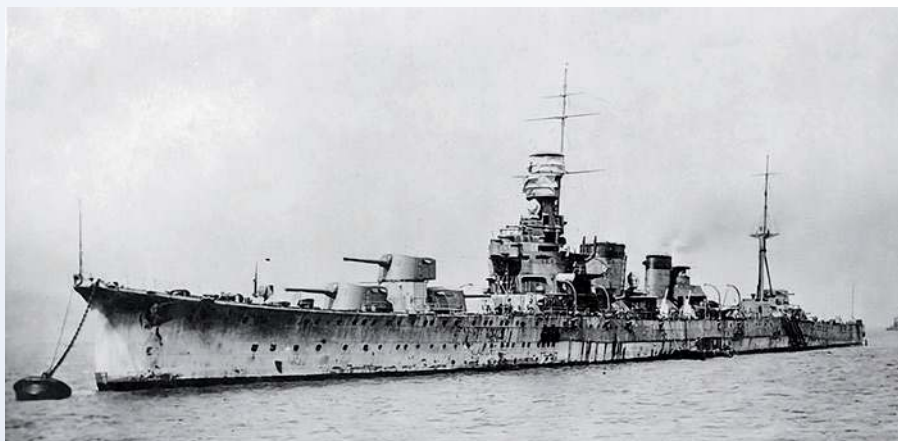
▲ Krążownik ciężki Kako niedługo po przyjęciu do służby. Widoczny układ artylerii głównej z pojedynczymi wieżami armat 200 mm, ustawionymi „piramidowo”. Można zauważyć też jasne płócienne pokrowce przykrywające najwyższe kondygnacje nadbudówki głównej, elementy systemu kontroli ognia oraz armaty przeciwlotnicze.
