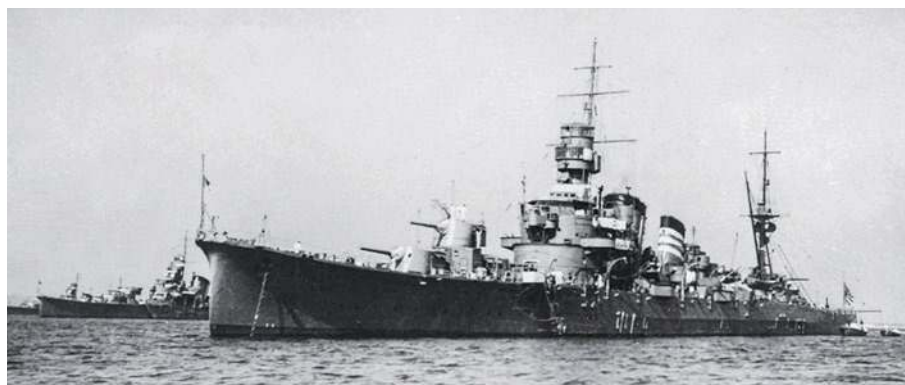
▲ Furutaka podczas postoju na kotwicy koło Shinagawy w Zatoce Tokijskiej w październiku 1935 r. Trzy pasy na kominie wskazują na pozycję trzeciego okrętu w 6 Dywizjonie. Za Furutaką widoczne są krążowniki Kinugasa i Aoba , należące do tego samego dywizjonu.
