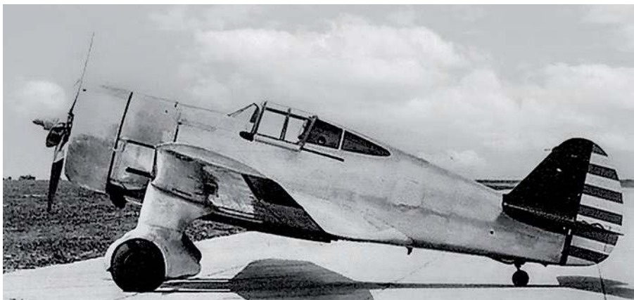
◀ Curtiss Hawk 75M widziany z lewej strony. Uważa się, że jest to pierwszy samolot tej wersji c/n 12625 sfotografowany w Buffalo przed przemalowaniem na olive drab 21 czerwca 1938 roku. Hawki 75M zamówione po wybuchu wojny zostały zmodyfikowane, co jednak pogorszyło osiągi w porównaniu do Hawka 75H (nazywanego Hawk Special ).
