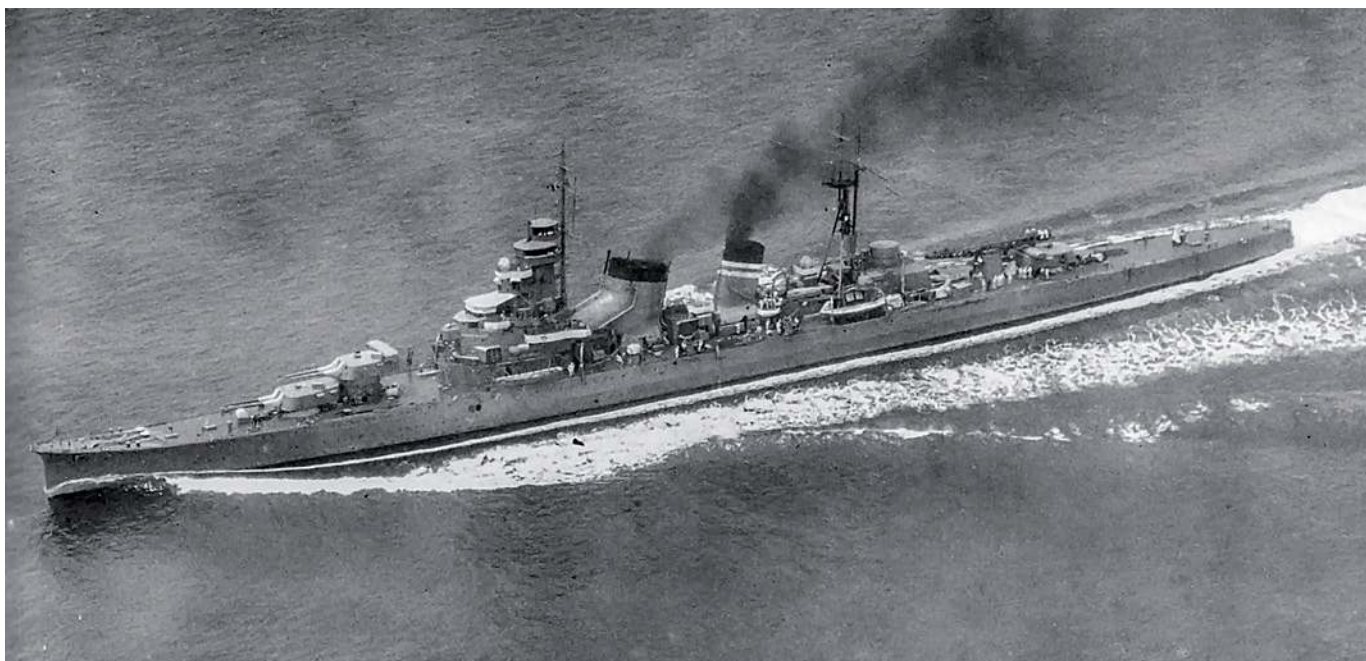
▼ Aoba widziana z samolotu, podczas marszu w latach 30. Dobrze widoczne szczegóły konstrukcji okrętu – wieże artylerii głównej, nadbudówki, kominy, maszty, pomocniczy director na rufowej nadbudówce i katapulta dla wodnosamolotów. Widać również płócienne zadaszenie pomostu kompasowego.
