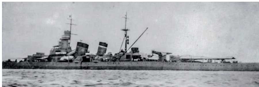
► Widok na śródkręcie krążownika Aoba w latach 30. Widoczna jest wieżyczka z pomocniczym directorem dla artylerii głównej zaraz za głównym masztem, a także znajdująca się pomiędzy nią a wieżą nr 3 katapulta dla wodnosamolotów.
