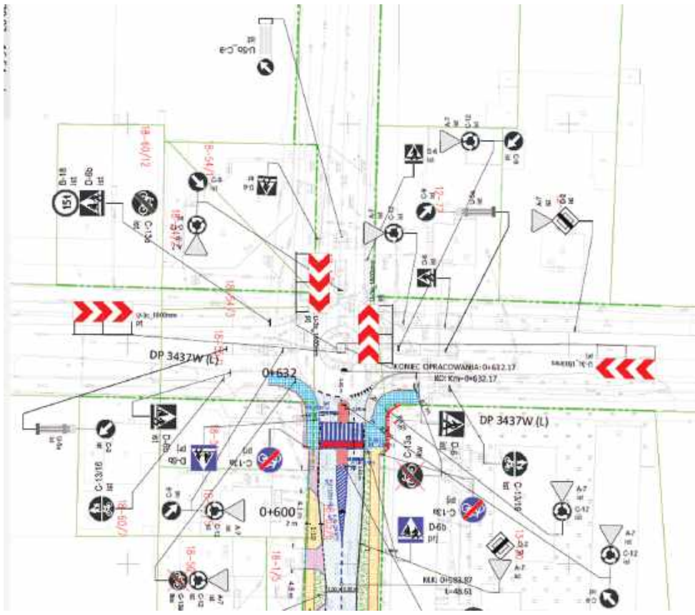
Projekt przebudowywanego ronda
