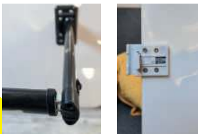
Sposób zmiany długości nogi stołu i zaczep blatu do szyny; długość podpory jest dobrana prawidłowo do funkcji jadalnej i sypialnej
