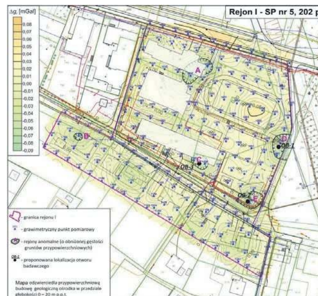
Wyniki badań mikrograwimetrycznych Rejonu I
