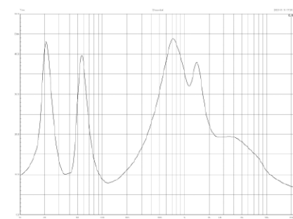
Rys. 5. Charakterystyka modułu impedancji.
