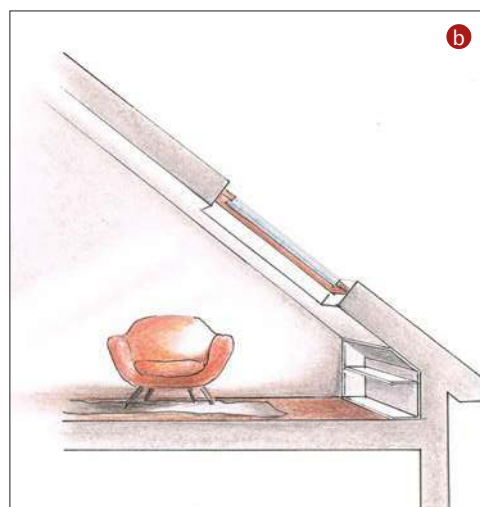
Do pełnego wykorzystania nadaje się tylko ta część poddasza, która ma od 1,9 m wysokości (a). Żeby przy ścianie ustawić meble, wystarczy 1,2 m (b).
