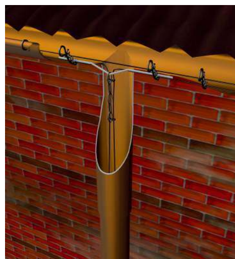
○ Kable w rurach i rynnach mocuje się pojedynczo lub podwójnie. ZAMEL
