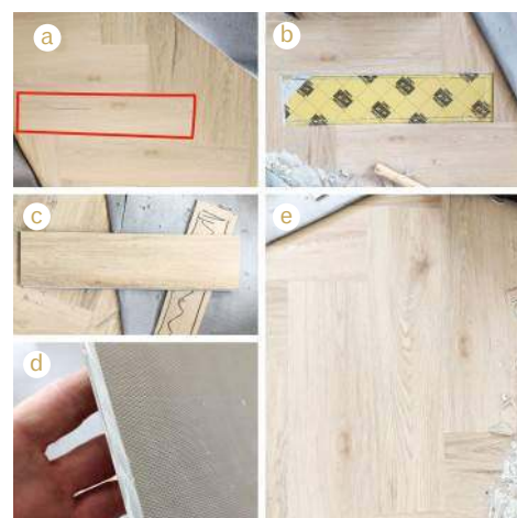
🔧 Wymiana panelu winylowego. Uszkodzony element do wymiany (a), wycięcie deski (b), nowy panel przygotowany do montażu (c), zbliżenie na fragment wyciętego zamka (d), gotowa podłoga (e). DECORA (ARBITON)
