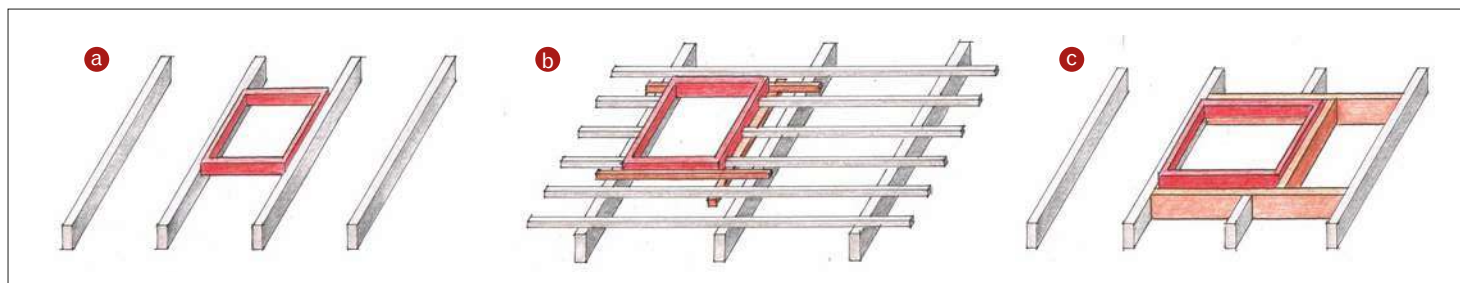
➊ Montaż okna połaciowego na krokwiach (a), łątach (b), wymianach (c).
