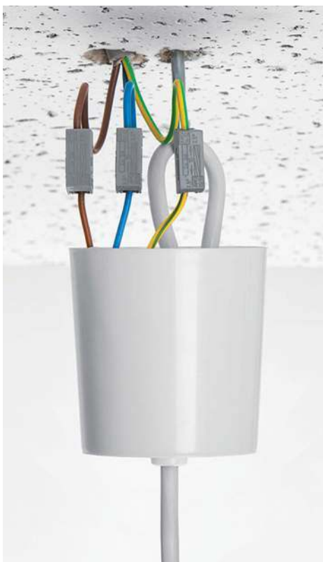
⚡ Szybkozłączki ułatwiają prace instalacyjne. WAGO ELWAG
