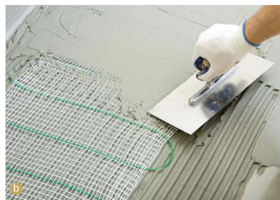
🔧 Wyrównywanie podłoża przed układaniem płytek (a BAUMIT), zatapianie mat grzewczych ogrzewania podłogowego (b CERESIT).
