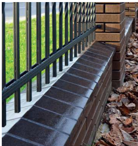
🔧 Trwałe ogrodzenie z cegły klinkierowej. Jego górną część można wykończyć ceglami kształtowymi. KLINKIER PRZYSUCHA
