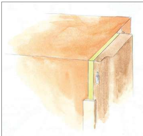
➤ Ościeżnice stałe najlepiej sprawdzają się w przypadku ścian o grubości 6–10 cm. Wymagają zastosowania listew maskujących (opasek) przytwierdzanych za pomocą kleju montażowego. Szczelinę między opaską a ścianą wypełnia się masą akrylową. POL-SKONE
