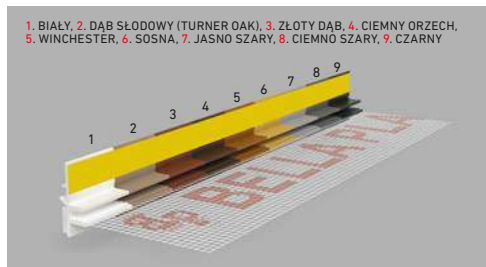
BP13 MIDI KOLOR LISTWY PRZYKLEPNE PVC KOLOROWE DYLACYJNE Z SIATKĄ I Z USZCZELKĄ
