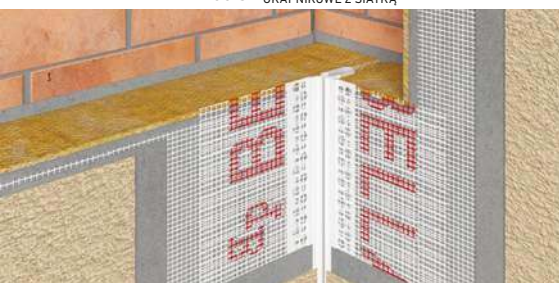
BP16 V LISTWA PVC DYLACYJNA TYPU „V” - KĄTOWA Z SIATKĄ
