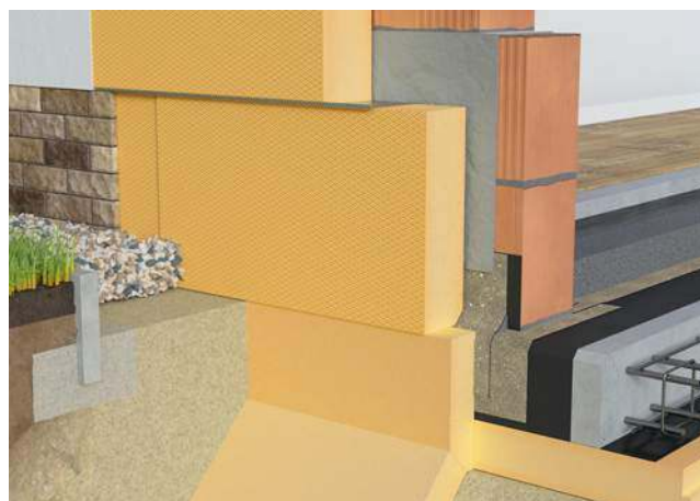
🔑 XPS w strefie cokołowej to dobry wybór. Tu wyzwaniem jest ewentualne zawilgocenie, a potem ciągłe zamarzanie i odmarzanie wody w materiale. SWISSPOR
