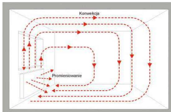
Sposoby rozprowadzania ciepła.
