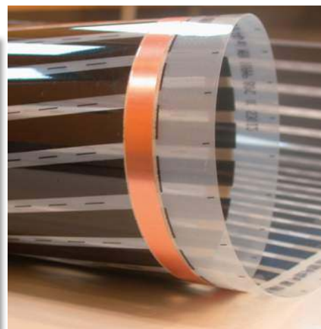
Folia grzejna do ogrzewania sufitowego, którą przykrywa się płytą gipsowo-kartonową może być alternatywą dla ogrzewania podłogowego. FENIX POLSKA
