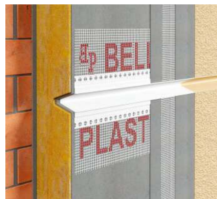
❶ Listwa z PVC do boniowania trójkątna – rąbek wklęsły. BELLA PLAST
