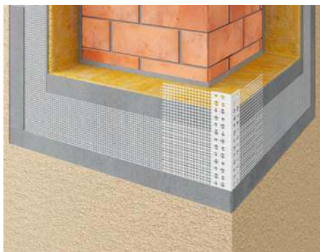
BP10 – kątownik PVC z siatką.
