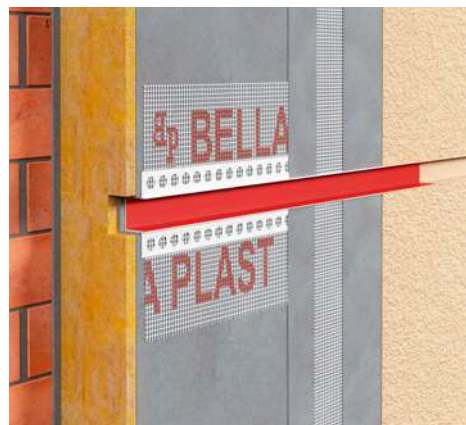
BP11 H2RS – listwa PVC do boniowania.
