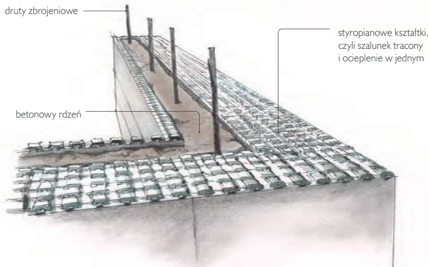
Ściana ze styropianowych kształtek.
