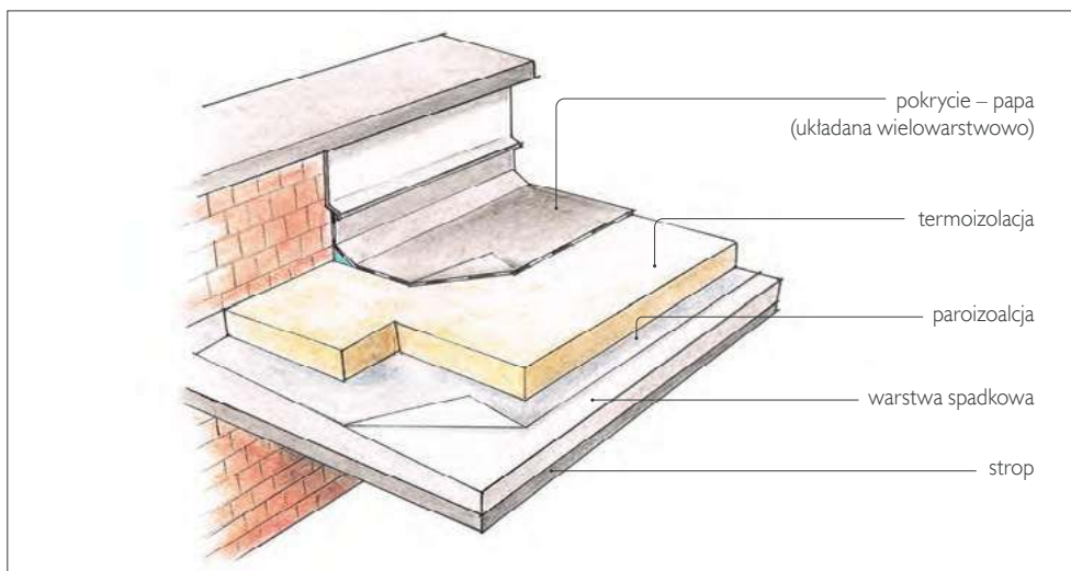
➤ Stropodach niewentylowany – w domach energooszczędnych ocieplenie powinno mieć przynajmniej 30 cm grubości.
