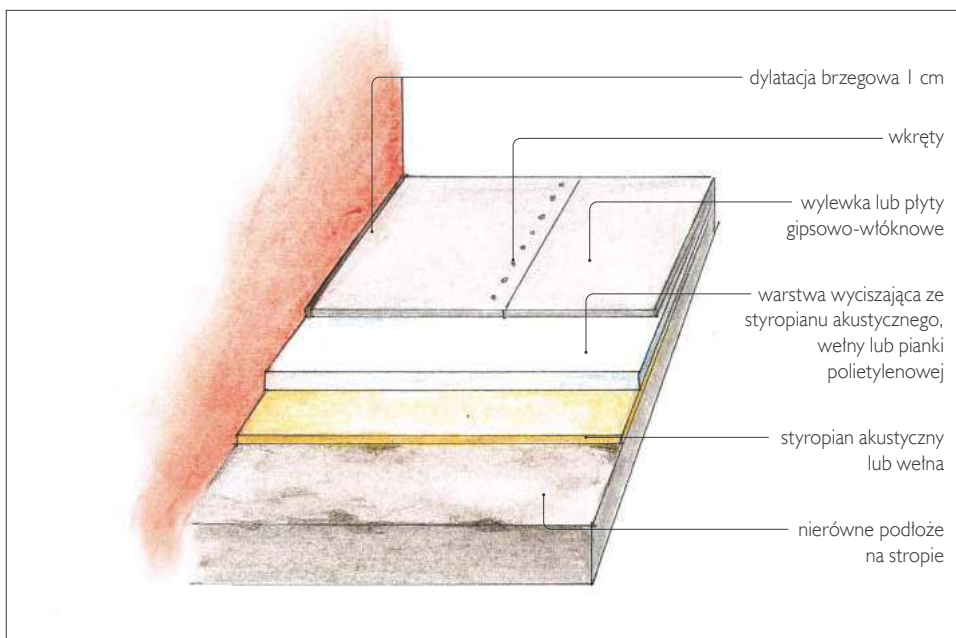
Podłoga na stropie żelbetowym.
