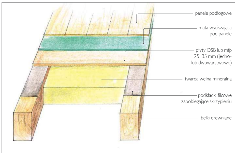
Podłoga na stropie drewnianym wykończona panelami.
