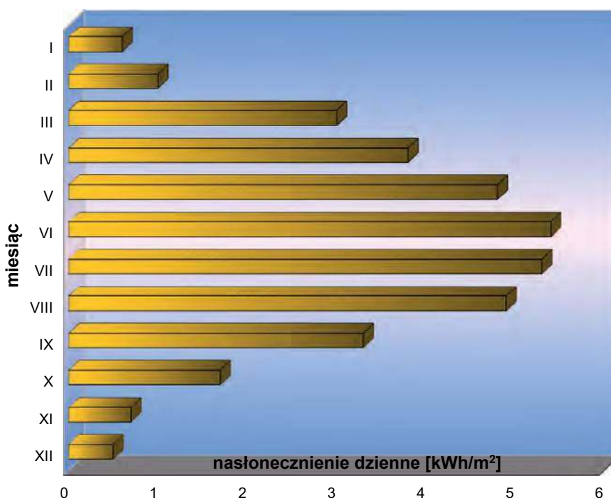
Nasłonecznienie dzienne 1 m 2 powierzchni – płaszczyzna o nachyleniu 45° (dane dla Warszawy)
