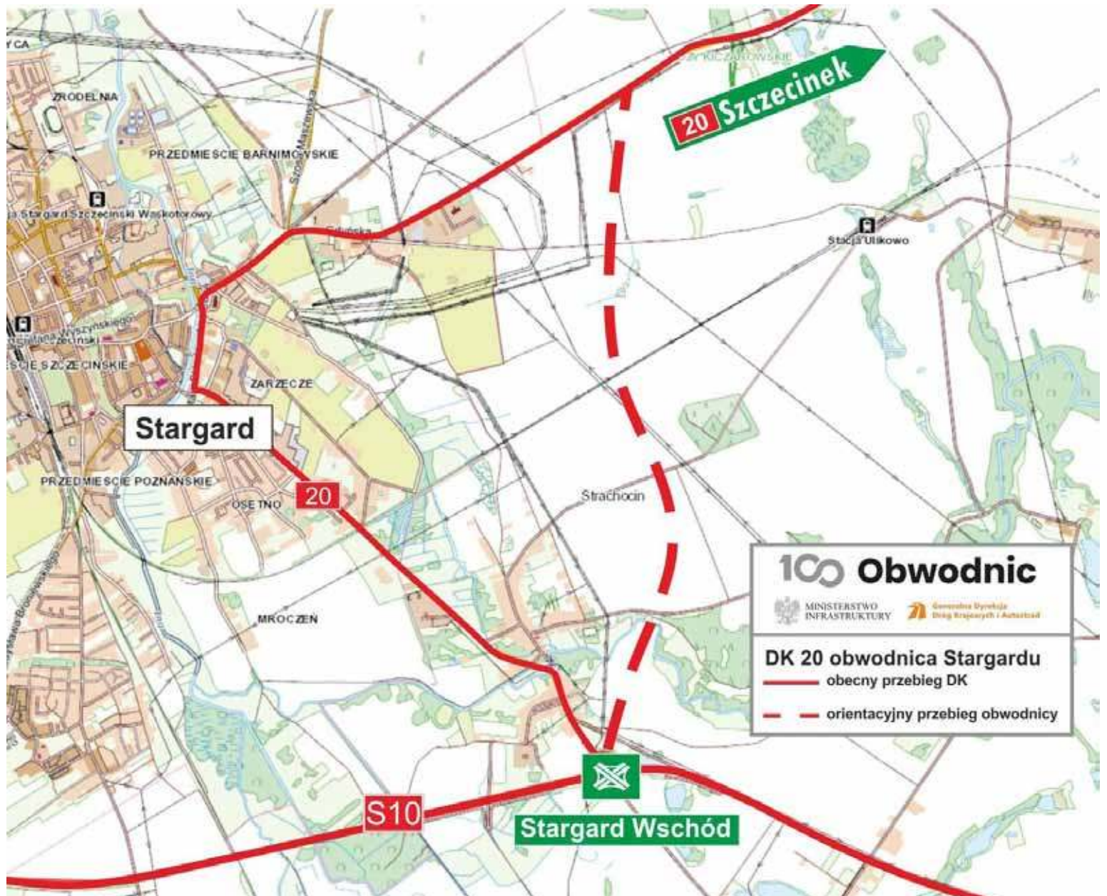
Orientacyjny plan DK nr 20 - obwodnicy Stargardu
