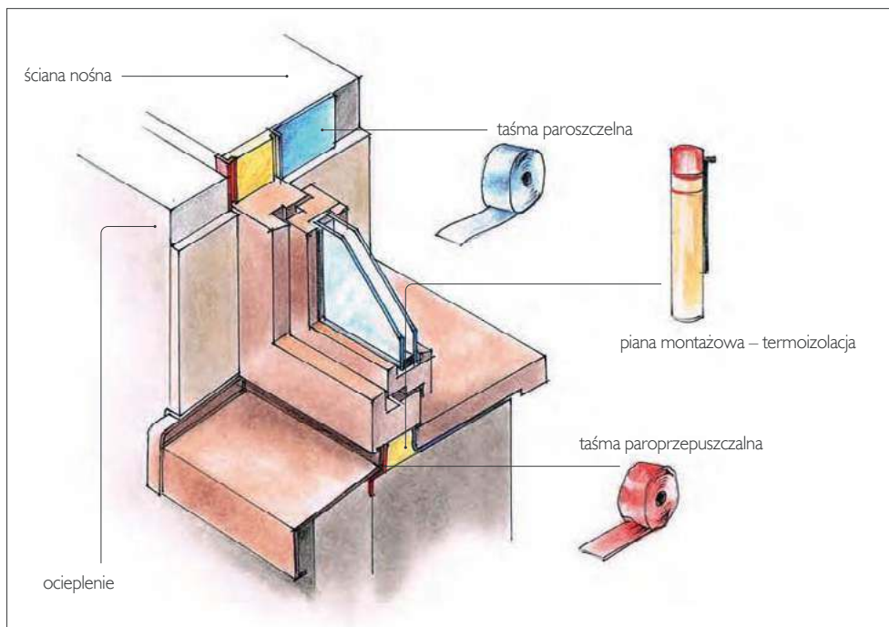
Elementy montażu warstwowego okna.
