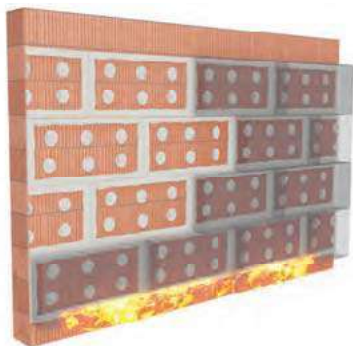
📌 Obwodowe pasy kleju zapobiegają rozprzestrzenianiu się ognia oraz ruchowi powietrza pomiędzy ociepleniem i murem. SWISSPOR
