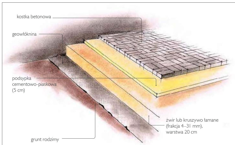
➤ Sposób wykonania tarasu na gruncie wykończonego kostką betonową.
