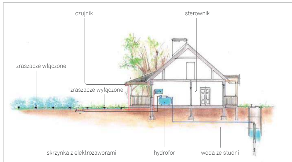
📌 Schemat systemu automatycznego nawadniania.
