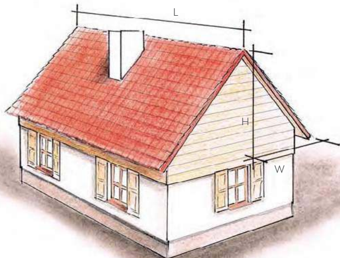
Wymiary niezbędne do wyznaczenia efektywnej powierzchni dachu.
