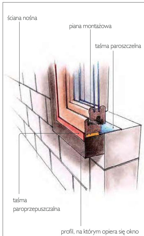
Montaż okna w warstwie ocieplenia
