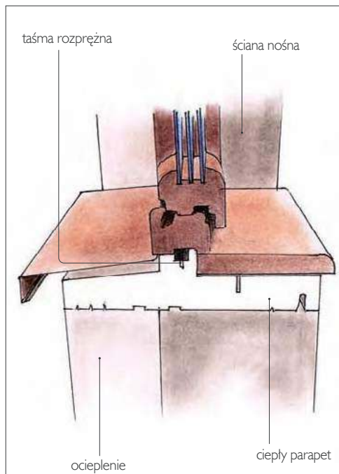
Sposób osadzenia ciepłego parapetu.
