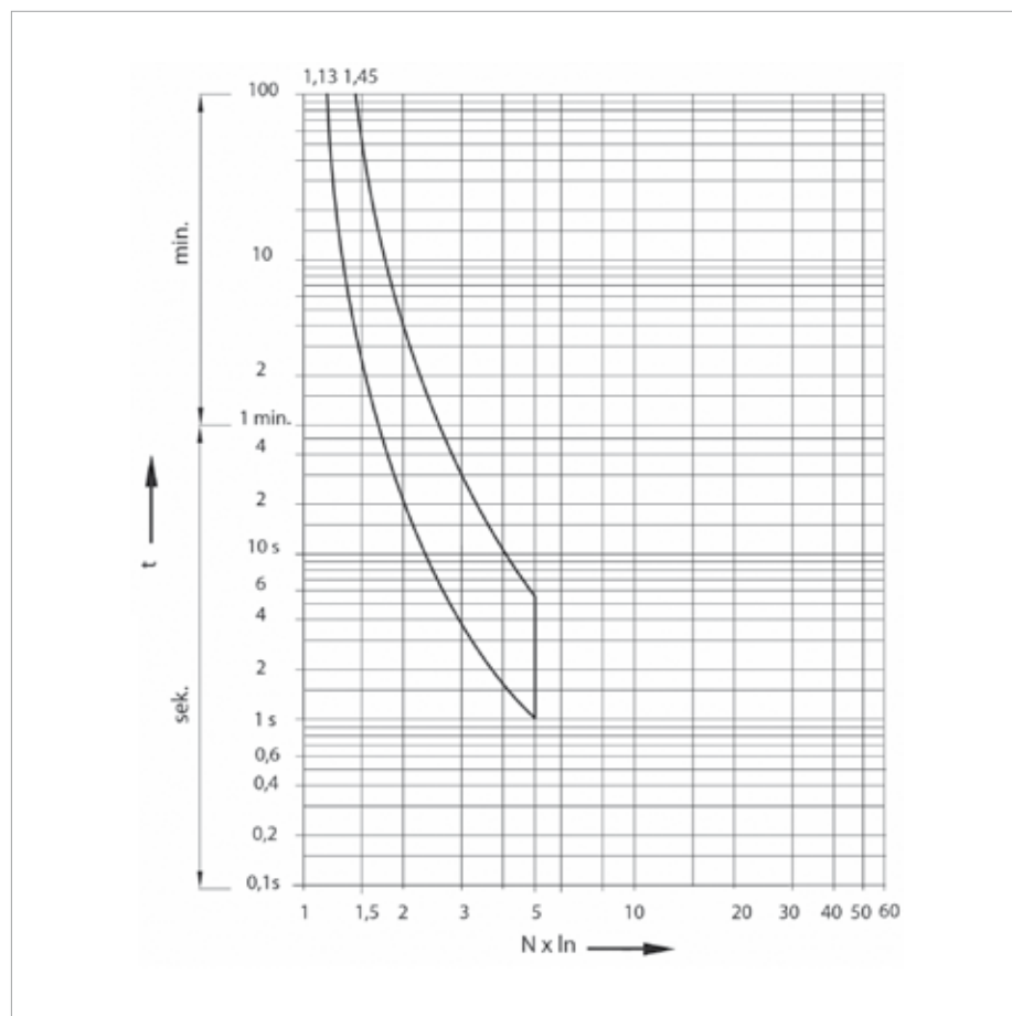
Rys. 4. Charakterystyka czasowo-prądowa t(I) ogranicznika mocy umownej ETIMAT T (bez członu zwarciovego)
