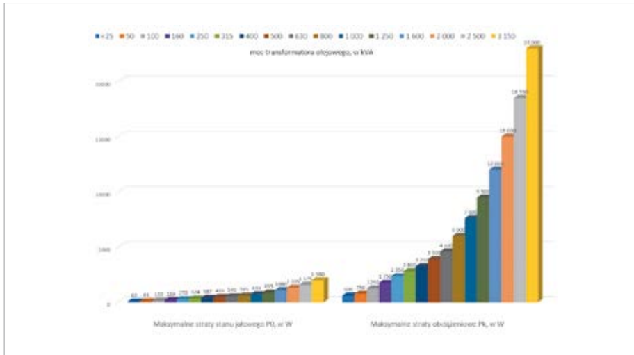
Rys. 1. Maksymalne straty obciążeniowe i maksymalne straty stanu jałowego dla trójfazowych olejowych transformatorów elektroenergetycznych o mocy znamionowej \leq 3150 kVA po 1 lipca 2021 r. [7]
