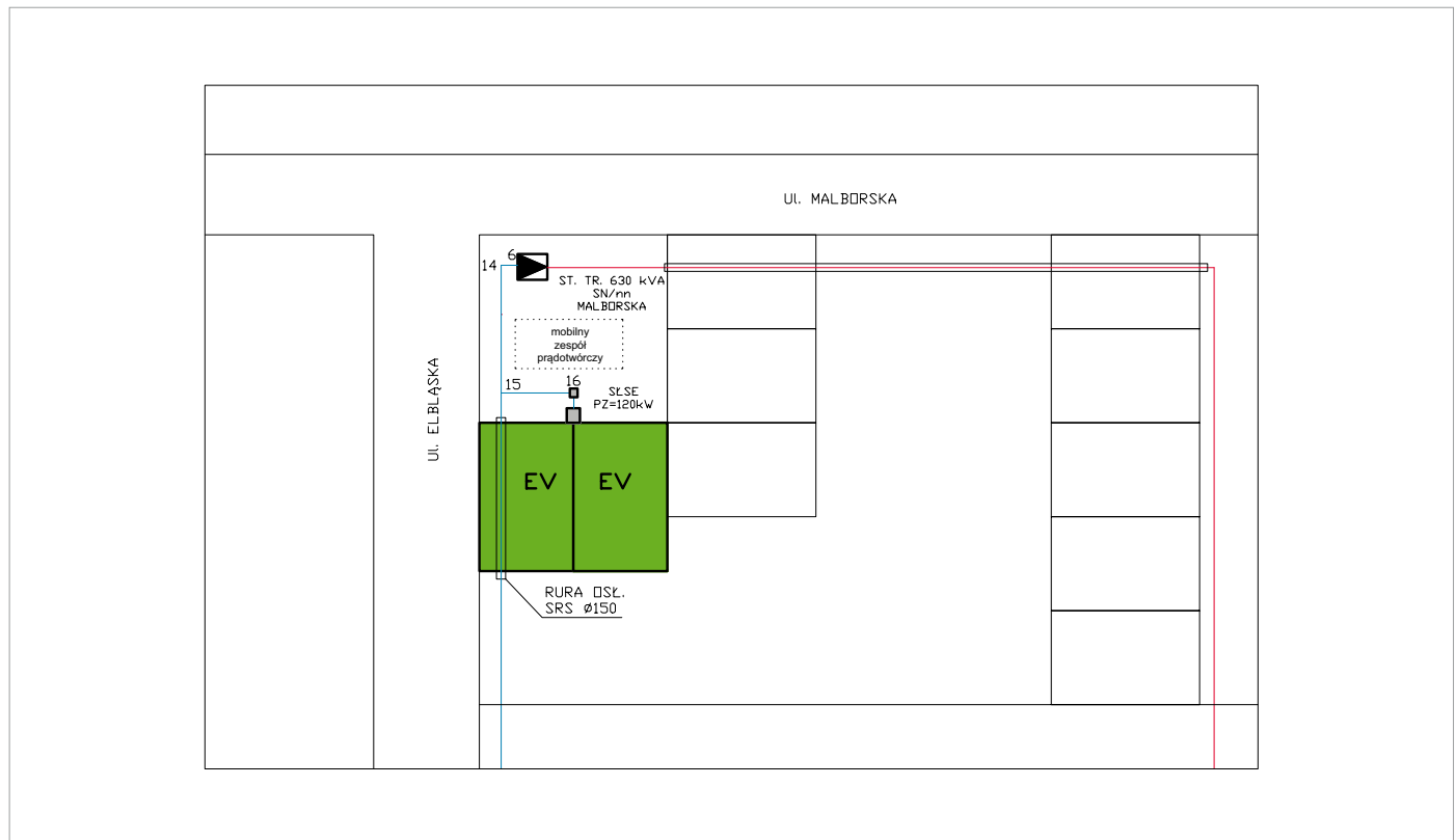
Rys. 1. Plan linii kablowych rys. J. Wiatr, M. Orzechowski
