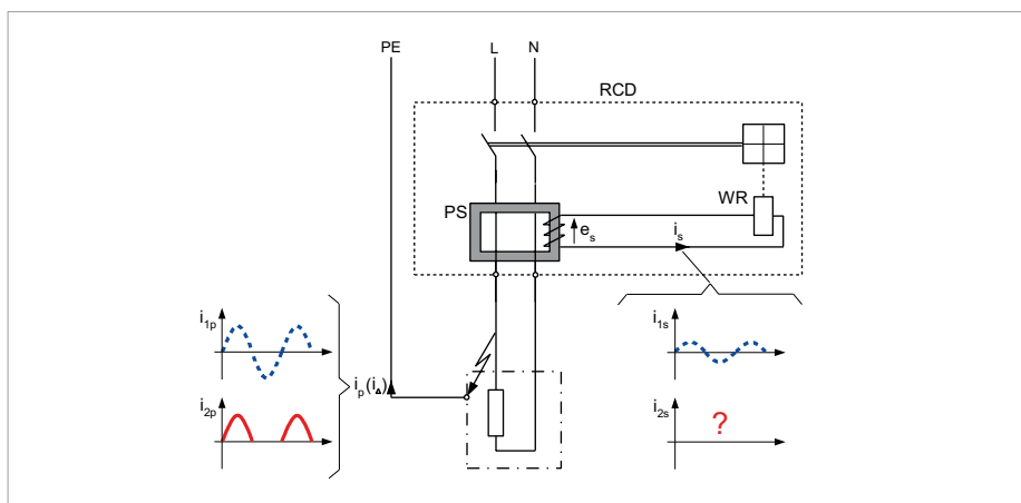
Rys. 1. Uproszczona struktura wyłącznika różnicowoprądowego (RCD) typu AC, gdzie: PS – przekładnik sumujący, WR – wyzwalacz różnicowy, i_p ( i_A ) – prąd pierwotny (różnicowy), i_s – prąd wtórny, e_s – napięcie indukowane w uzwojeniu wtórnym przekładnika PS rys. S. Czapp
