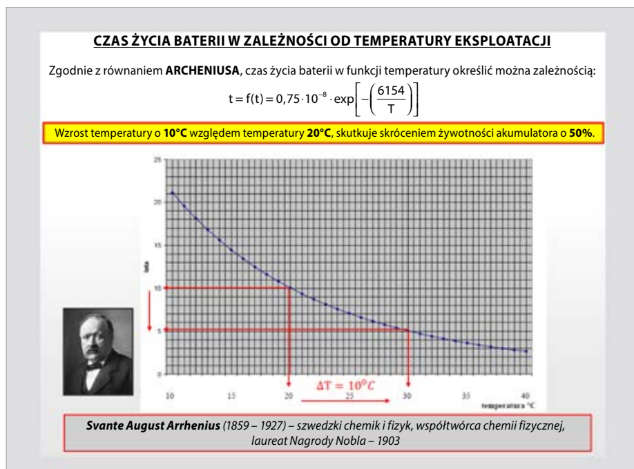
Fot. 4. Zależność żywotności akumulatora wg Svante A. Arrheniusa, w funkcji temperatury [10]
