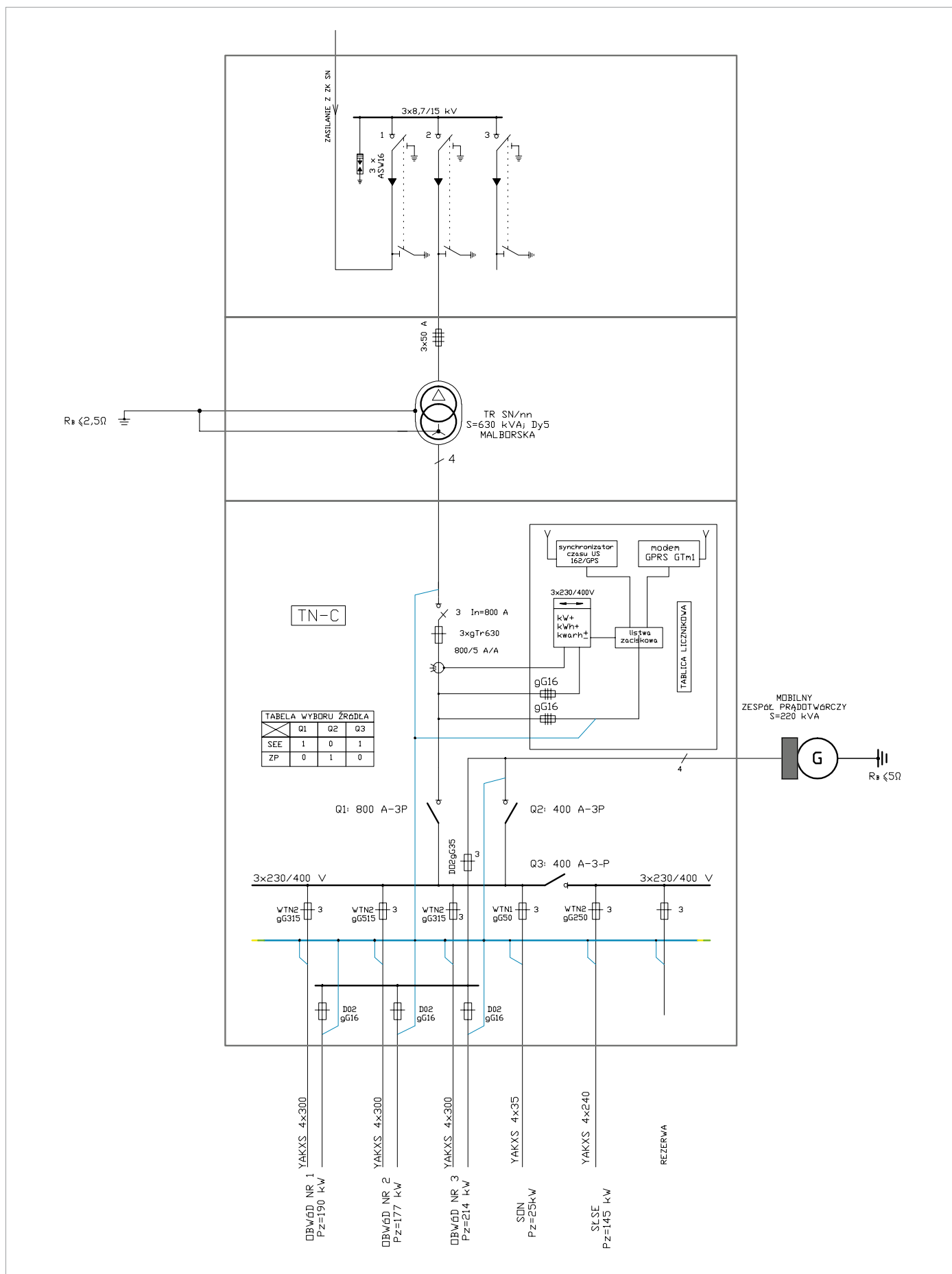
Rys. 2. Schemat stacji transformatorowej, zasilającej SŁSF rys. J. Wiatr, M. Orzechowski
