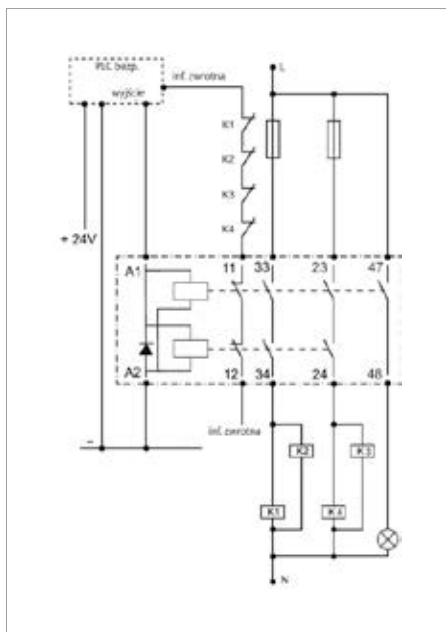
Rys. 2. Redundancja w przekaźniku Finder 75.43
