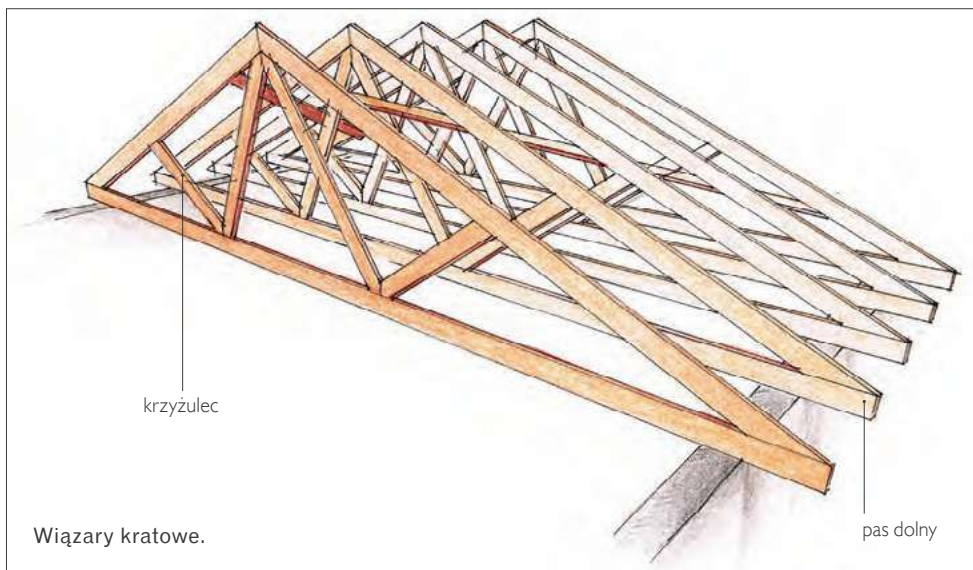
🔧 Wiązary wykonuje się nie na budowie, a w zakładzie produkcyjnym. Jedną z ich największych zalet jest bardzo szybki montaż – specjaliści mogą się z nim uporać nawet w jeden dzień. WIĄZARY BURKIETOWICZ
