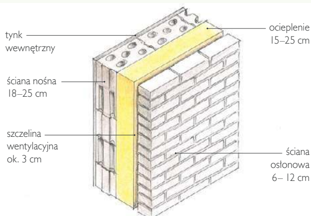
Trójwarstwowa ściana z z silikatów ocieplonych wełną mineralną.
