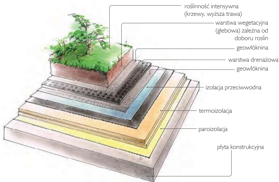
❗ Układ warstw zielonego dachu z roślinnością intensywną.
