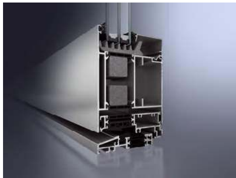
❶ Ciepły profil aluminiowy to dwa kształtowniki z metalu, połączone termiczną wkładką z tworzywa. SCHÜCO
