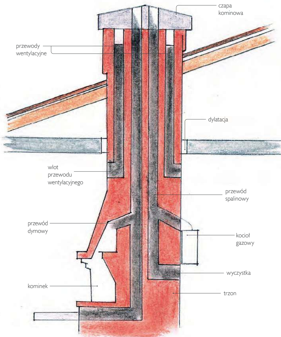
📍 Schemat rozmieszczenia w kominie kanałów wentylacyjnych, dymowych i spalinowych.
