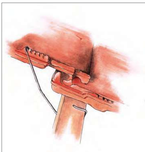
❗ Mocowanie dachówek za pomocą specjalnych klamerek.
