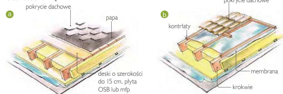
ⓘ Podkład w formie deskowania (a) i ołacenia (b).
