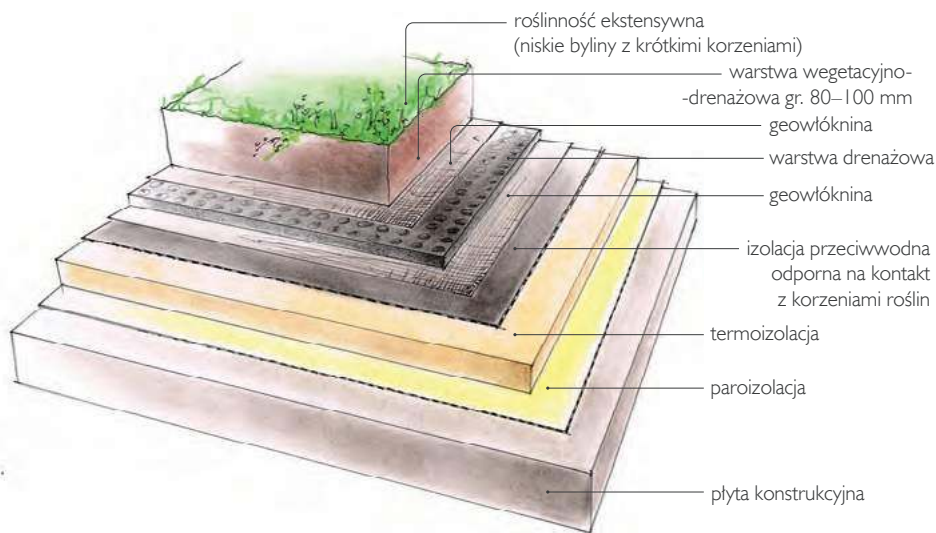
❗ Układ warstw zielonego dachu z roślinnością ekstensywną.
