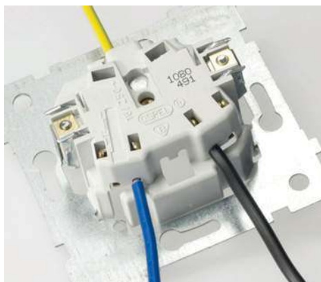
🔌 W obwodach gniazd stosuje się obecnie 3-żyłowe przewody miedziane o przekroju 3 \times 2,5 \text{ mm}^2 . OSPEL
