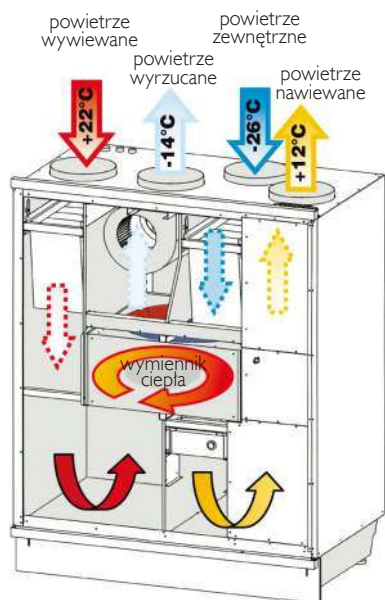
🔹 Zasada działania centrali z wymiennikiem ciepła. IGLOTECH
