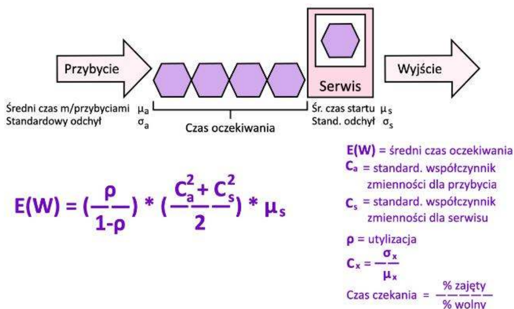
Rys. 6 Prawo Kingmana
