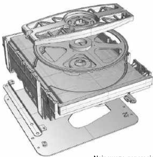
Najnowsza generacja napędu VRDS opiera się na dawnych założeniach; płyta jest stabilizowana za pomocą masywnego, górnego krążka.
