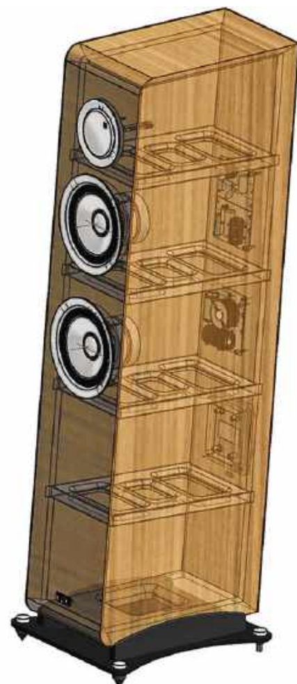
Obydwa głośniki pracują we wspólnej komorze, obudowa jest wzmocniona czterema wieńcami.
