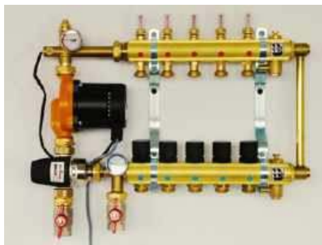
🔧 Rozdzielacz z termostatycznym zaworem mieszającym umożliwia obniżenie temperatury zasilania pętli podłogowych. TEECE
