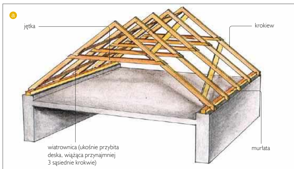
📍 📍 Podstawowe konstrukcje ciesielskie: krokwiowo-jętkowa (a) i płatwiowo-kleszczowa (b).
