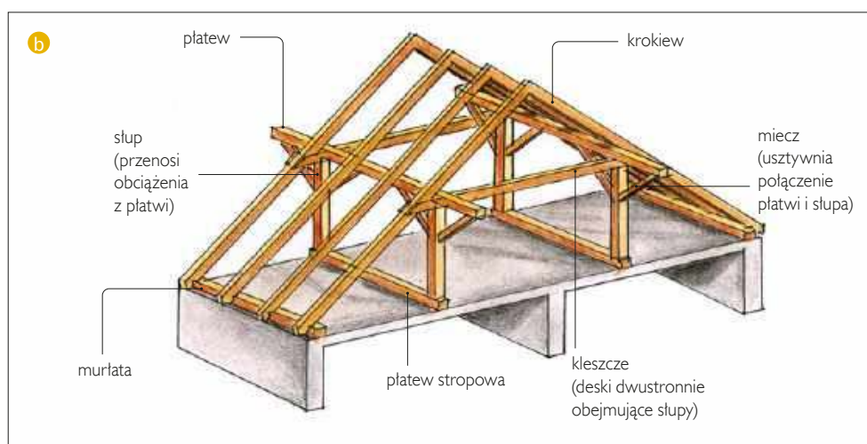
📍 📍 Podstawowe konstrukcje ciesielskie: krokwiowo-jętkowa (a) i płatwiowo-kleszczowa (b).
