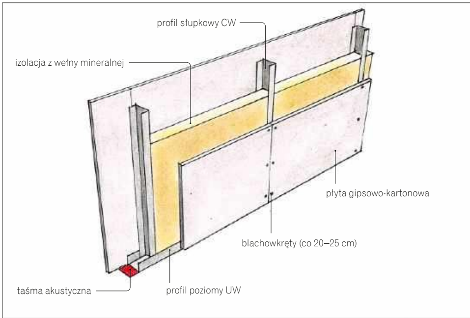
❶ Ściana działowa z jednowarstwowym poszyciem z płyt g-k.
