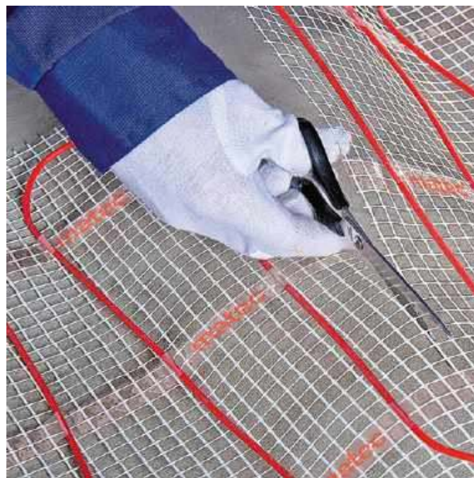
🔧 Ogrzewanie podłogowe montuje się na równym podłożu, które musi być zaizolowane termicznie. ZAMEL
