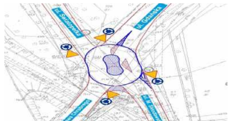
GDDKiA poinformowała, że na jezdni żółtymi liniami zaznaczy środkową wyspę ronda oraz wprowadzi odpowiednie znaki pionowe
