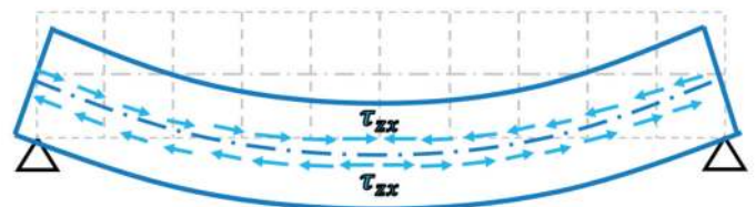
Rys. 6. Naprężenia styczne rozwarstwiający w połowie wysokości belki
