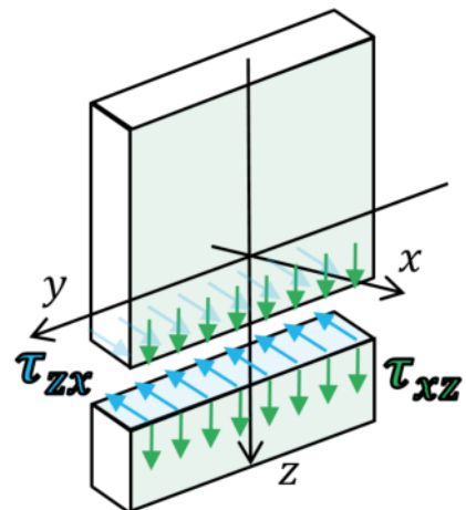
Rys. 5. Naprężenia styczne – składowe poziome (rozwarstwiający)
