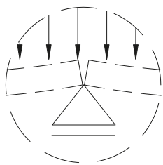
Rys. 2. Schemat ugięcia i skrócenia przeseł belki w wyniku obciążenia parciem mieszanki
