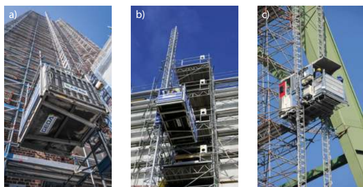
Fot. 4. Platformy transportowe GEDA:
