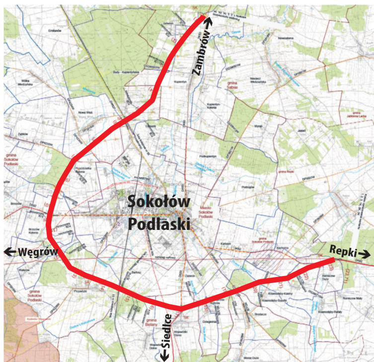
Jeden z planowanych wariantów obwodnicy Sokołowa Podl.
