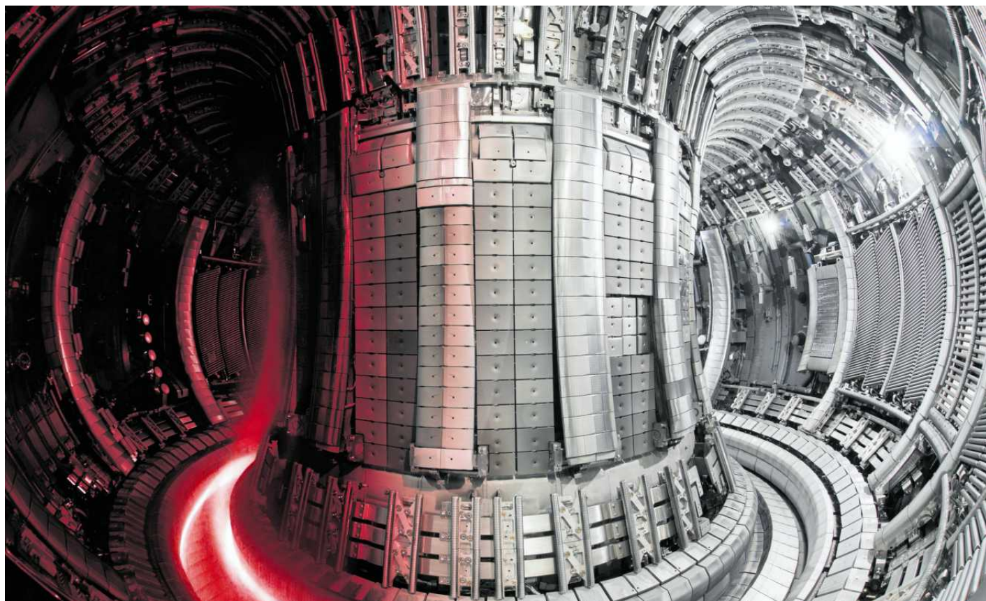
• Rozpalona plazma w komorze tokamaka JET FOT. UKAEA
