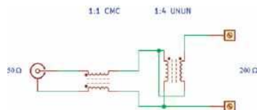
Rys. 10. Schemat obwodu dopasowującego do anteny LPi
