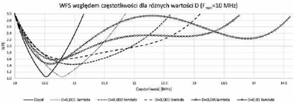
Rys. 3. Porównanie współczynnika fali stojącej WFS anten LPi o różnej wartości wymiaru D oraz dipola półfalowego. \lambda jest to długość fali najniższej częstotliwości pracy F_{min} , w tym przypadku – 30 m dla 10 MHz
