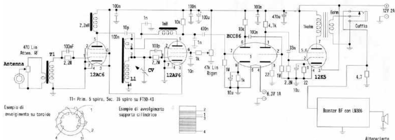
Rys. 5. Schemat ideowy reakcyjnego odbiornika na lampach
