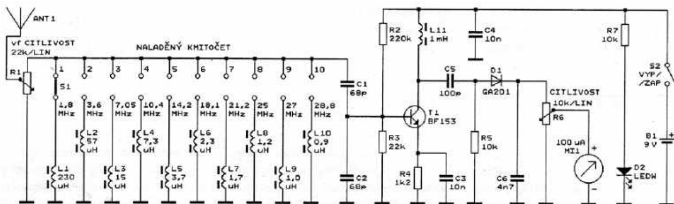
Rys. 2. Schemat ideowy wskaźnika pola EM
