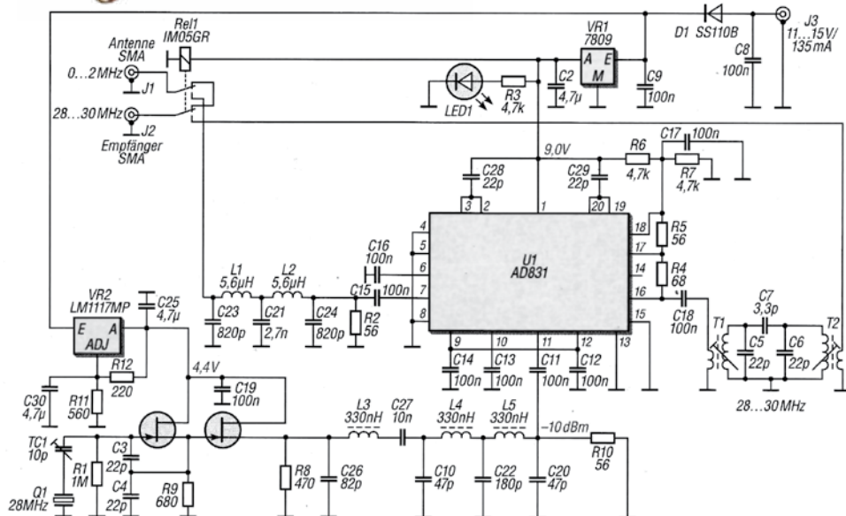
Rys. 1. Schemat ideowy konwertera LW UC-1S
