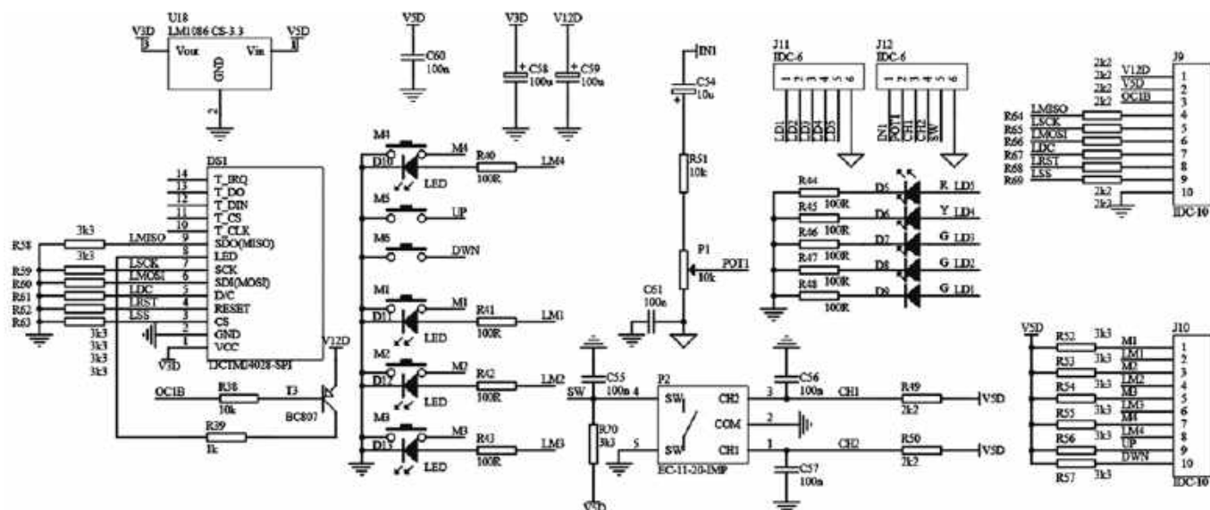
Rys. 2. Schemat przedniego panelu aktywnego głośnika
