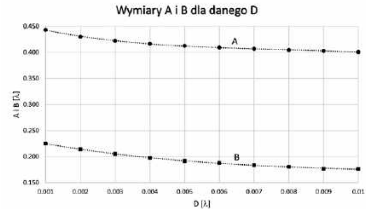
Rys. 6. Nomogram do wyznaczania wymiarów A i B przy znanym wymiarze D . Wszystkie wymiary są wyrażone w długości fali \lambda dla najniższej częstotliwości pracy anteny F_{min}
