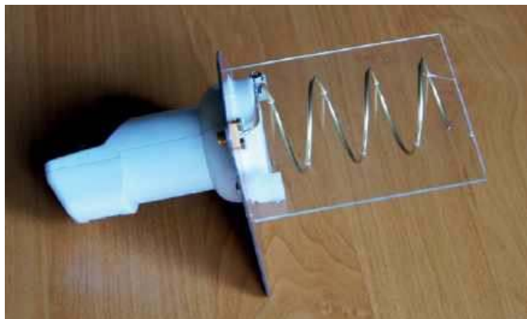
Fot. 3. Konwerter LNB z nadawczą anteną helikalną
