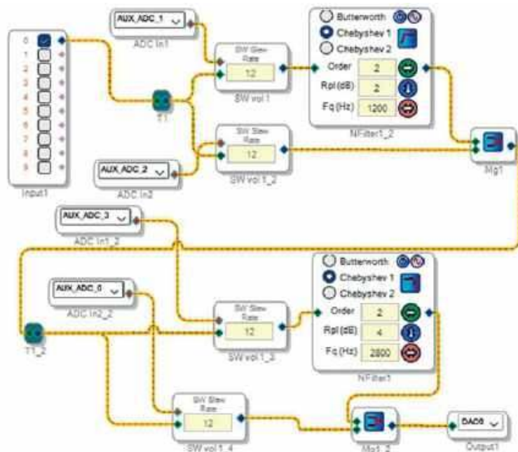
Rys. 1. Przykładowy projekt realizacji dwóch filtrów
