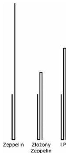
Rys. 2. Porównanie anteny LPi z anteną Zeppelin złożoną w pół
