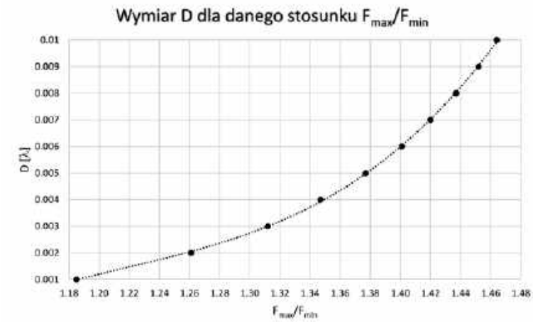
Rys. 5. Nomogram do wyznaczania wymiaru D anteny LPi. D jest wyrażone w długości fali \lambda w najniższej częstotliwości pracy anteny, to jest F_{min}
