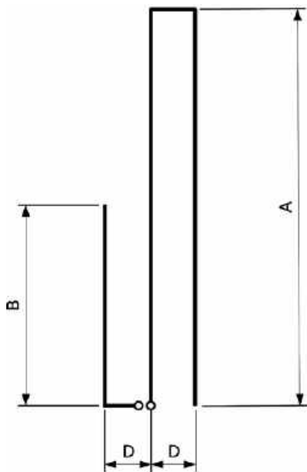
Rys. 1. Widok anteny LPi. Uwaga, rysunek nie zachowuje proporcji – w rzeczywistości pionowe przewody są umieszczone znacznie bliżej siebie niż na rysunku. Antena jest zasilana między „literą L” a „literą Pi”
