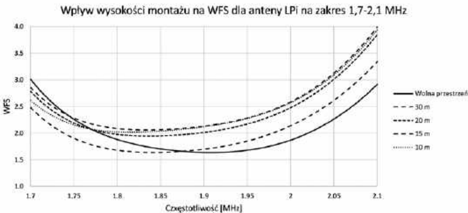
Rys. 7. Wpływ wysokości instalacji poziomo zawieszanej anteny LPi na jej WFS w paśmie 160 m
