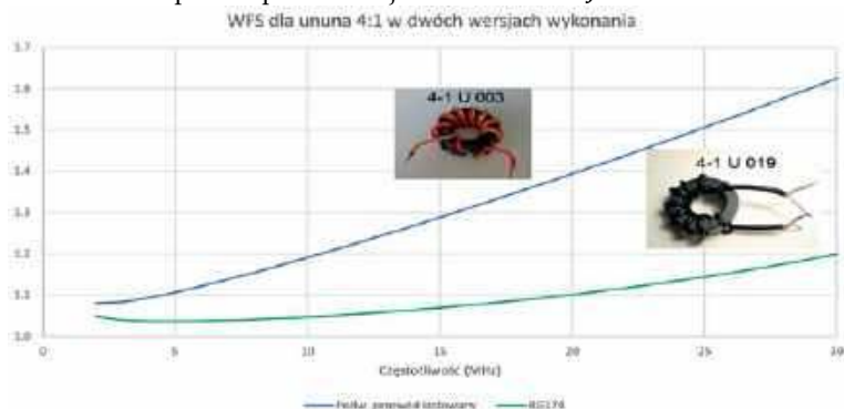
Rys. 13. Wykresy WFS dla dwóch wersji ununa 4:1
