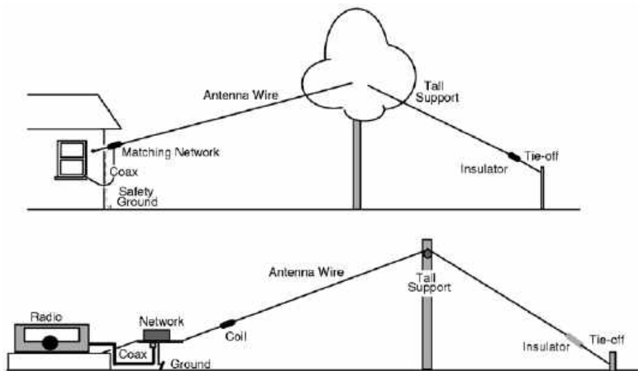
Typowe konfiguracje montażu anteny: powyżej – w warunkach domowych, poniżej – w terenie
