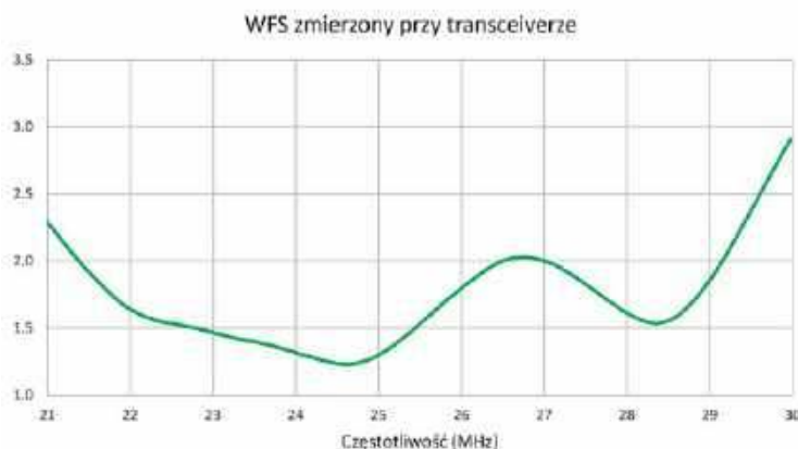
Rys. 12. WFS zmierzony przy transceiverze w całym zakresie częstotliwości pracy. Antena połączona z transceiverem niskostratnym kablem typu RF5 o długości 22 m
