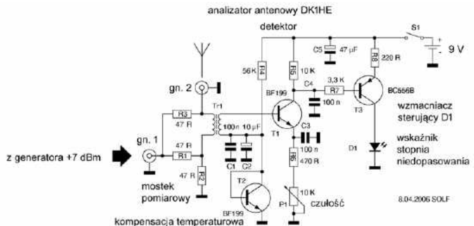
Rys. 1. Schemat ideowy analizatora antenowego DK1HE
