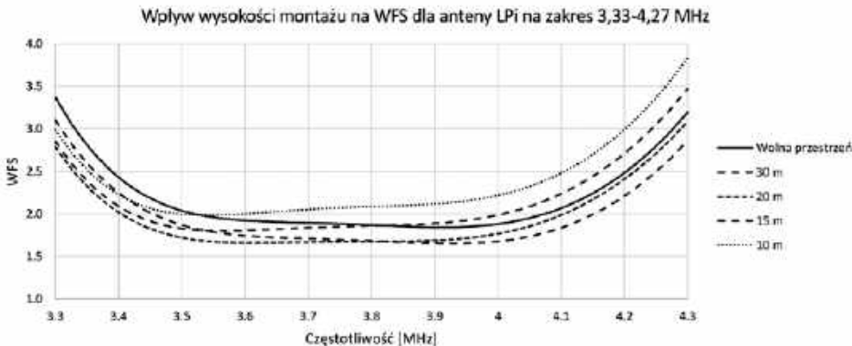
Rys. 8. Wpływ wysokości instalacji poziomo zawieszanej anteny LPi na jej WFS w paśmie 80 m
