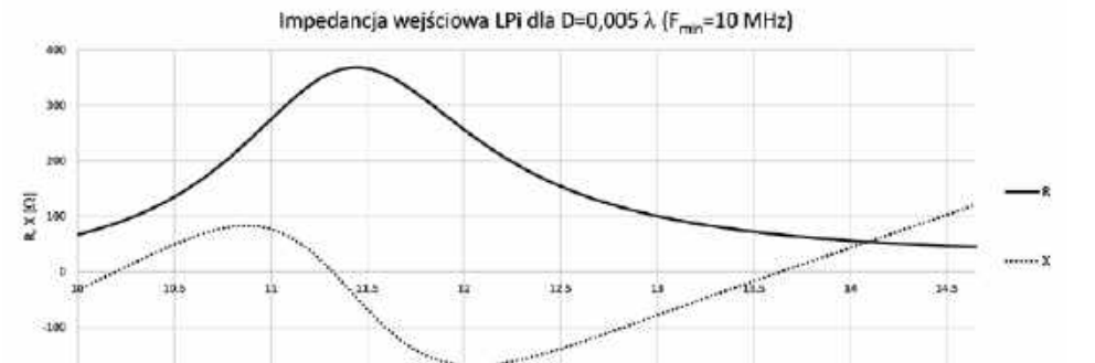
Rys. 4. Zależność impedancji wejściowej anteny LPi od częstotliwości
