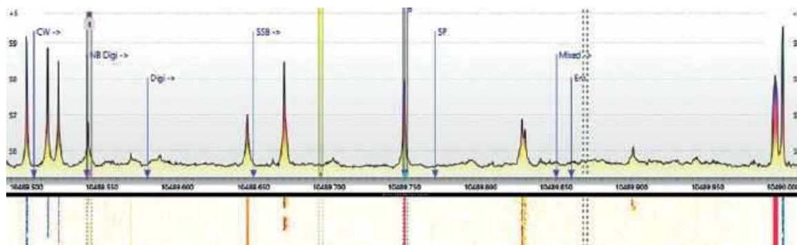
Rys. 2. Widmo odbiornika w programie SDR Console
