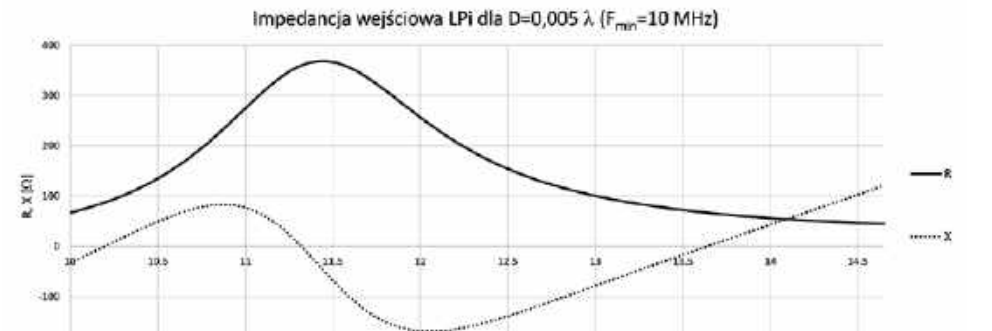
Rys. 4. Zależność impedancji wejściowej anteny LPi od częstotliwości
