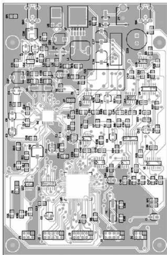
Rys. 5. Widok rozmieszczenia elementów na płytce drukowanej głośnika aktywnego
