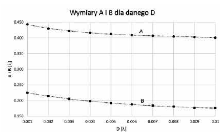
Rys. 6. Nomogram do wyznaczania wymiarów A i B przy znanym wymiarze D . Wszystkie wymiary są wyrażone w długości fali \lambda dla najniższej częstotliwości pracy anteny F_{min}
