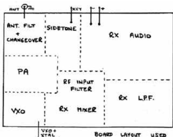
Rys. 4. Szkic rozmieszczenia poszczególnych bloków transceivera
