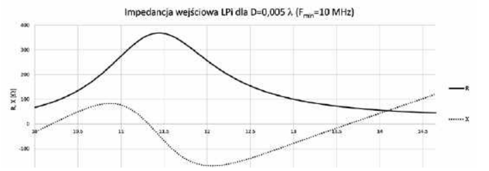
Rys. 4. Zależność impedancji wejściowej anteny LPi od częstotliwości
