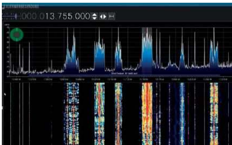
Rys. 5. Widmo stacji radiofonicznych AM
