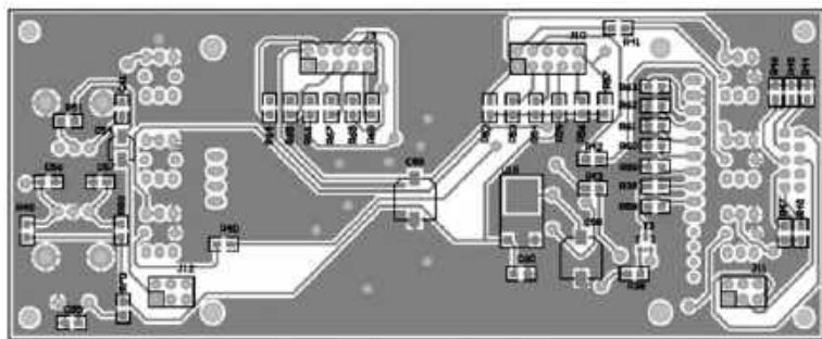
Rys. 4. Widok płytki drukowanej panelu przedniego od strony elementów SMD
