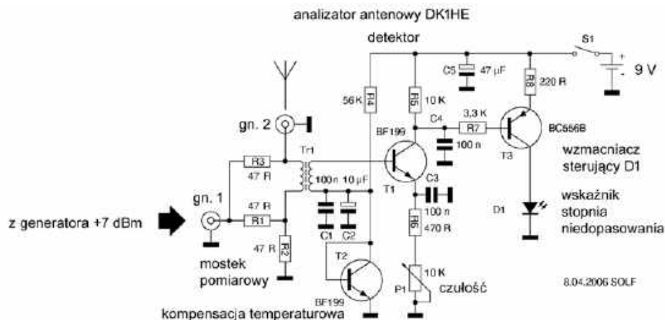
Rys. 1. Schemat ideowy analizatora antenowego DK1HE
