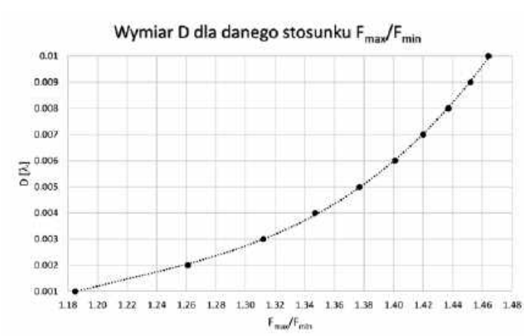
Rys. 5. Nomogram do wyznaczania wymiaru D anteny LPi. D jest wyrażone w długości fali \lambda w najniższej częstotliwości pracy anteny, to jest F_{min}
