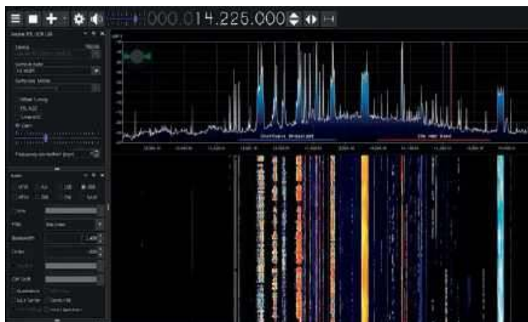
Rys. 3. Wskaźniki widma i wodospadoły w trakcie odbioru
