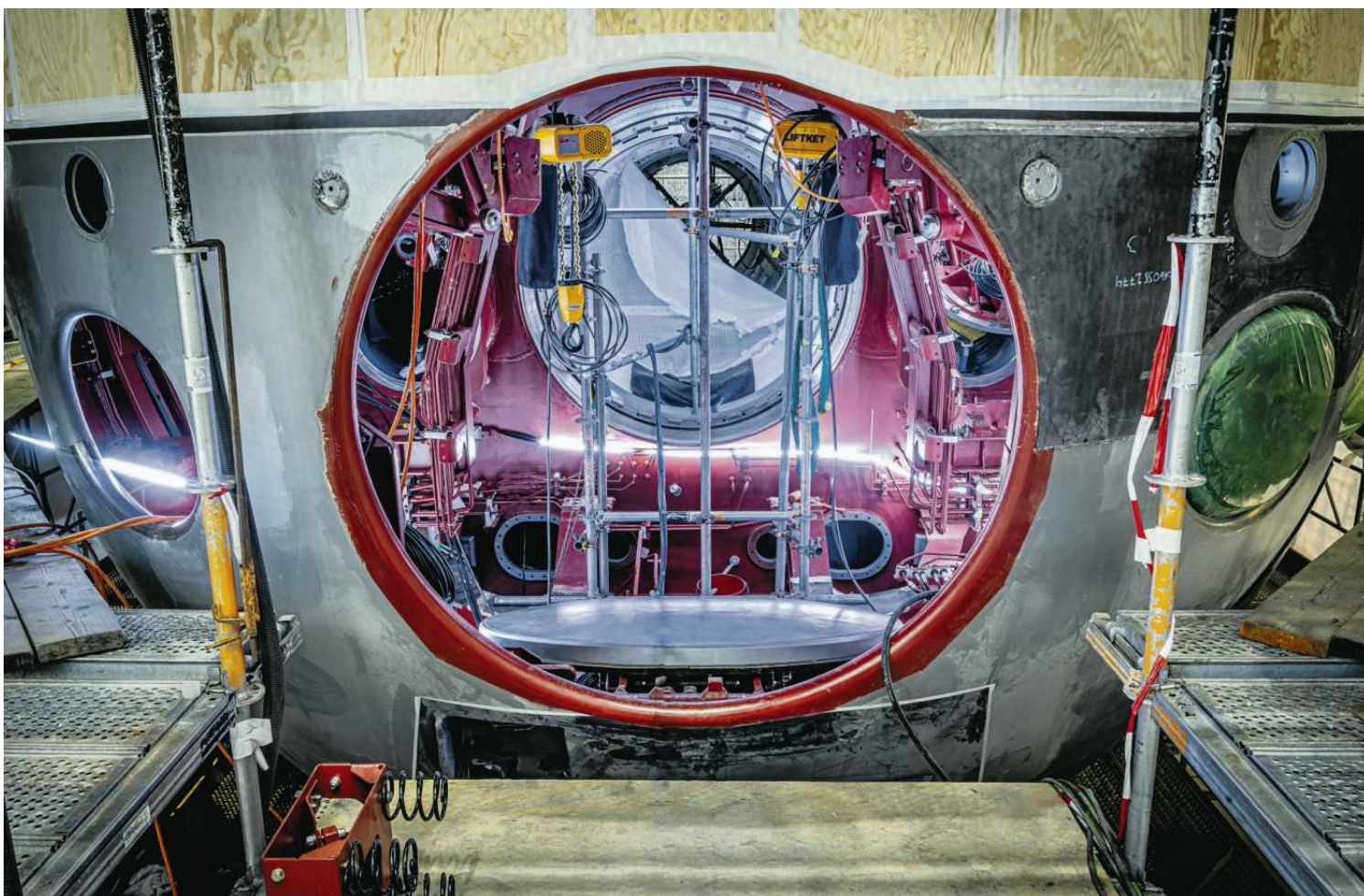
• Produkcja okrętów podwodnych A26 w stoczni Saab Naval w szwedzkiej Karlskronie FOT. GLENN PETTERSSON/SAAB KOCKUMS
