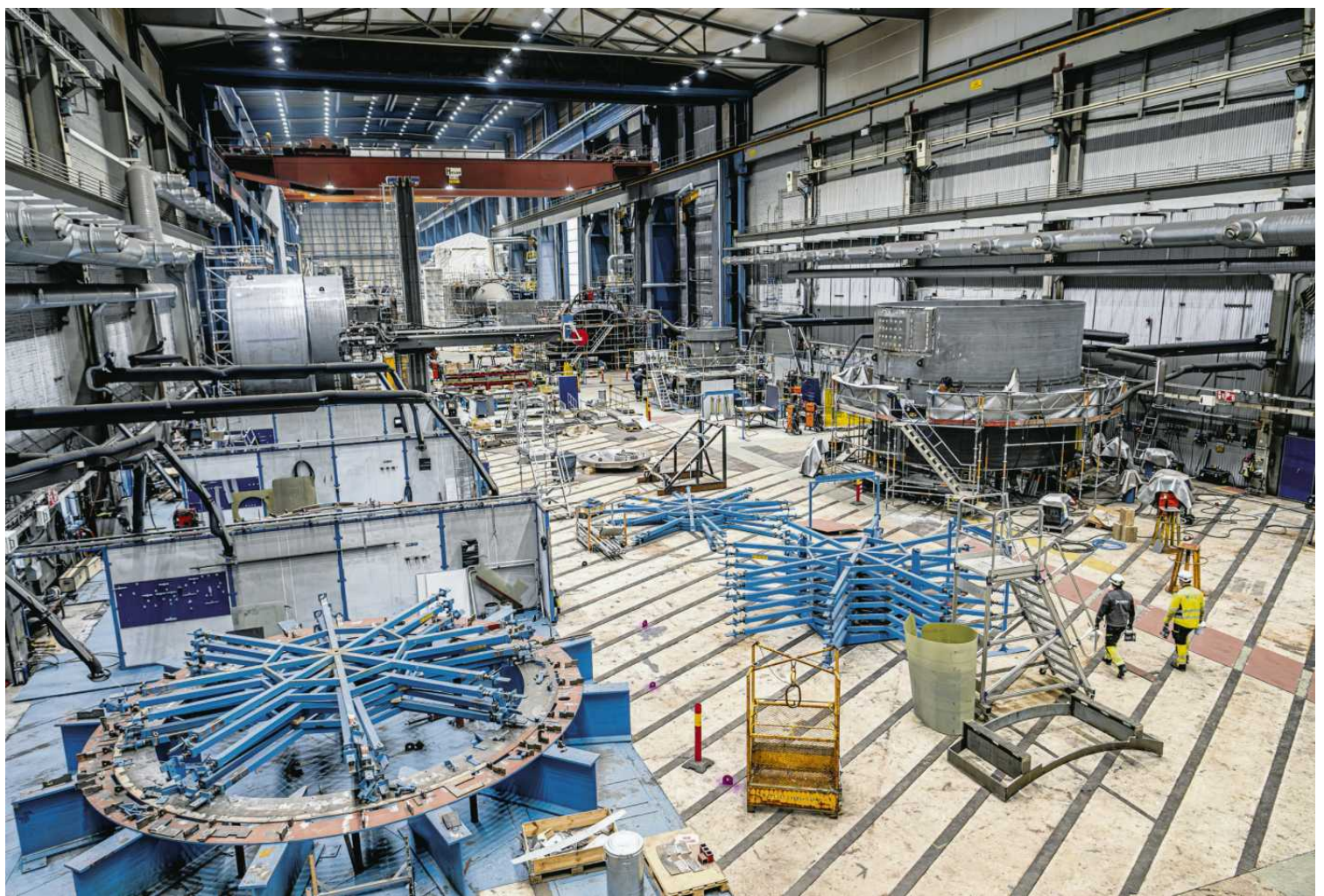
• Produkcja okrętów podwodnych A26 w stoczni Saab Naval w szwedzkiej Karlskronie FOT. GLENN PETERSSON/SAAB KOCKUMS
