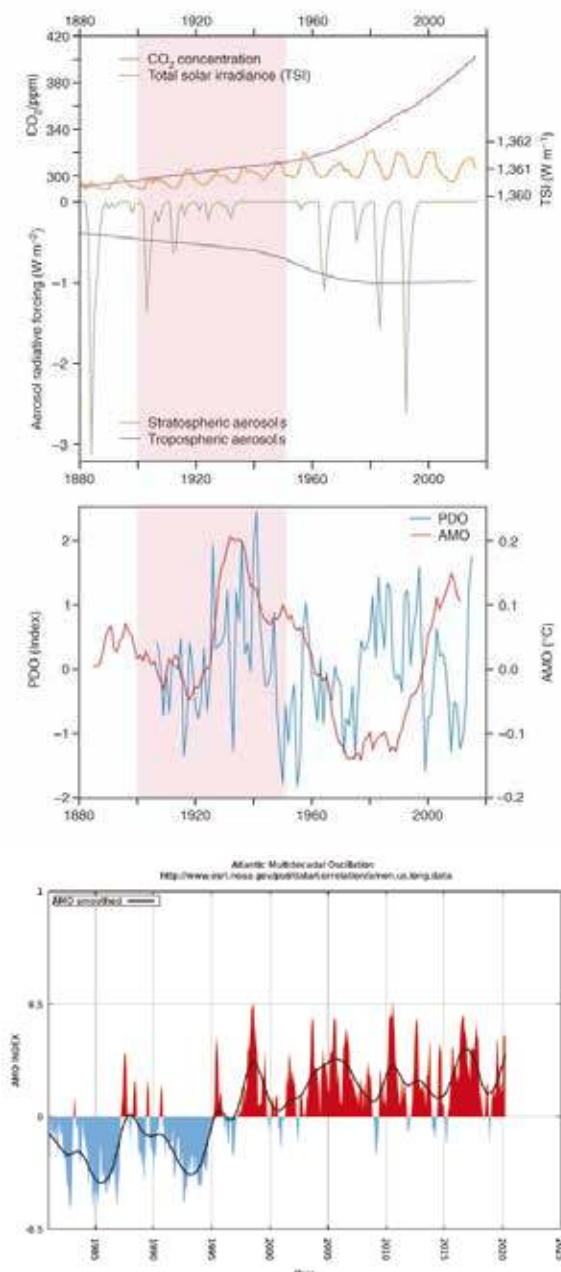
Rys. 3. Zmiany w kilku wymuszeniach zewnętrznych klimatycznych w ETCW (Wczesne Ocieplenie Dwudziestego Wieku). Obok jest aktualizacja zmian AMO do 2020 r. Źródło: Hegerl et. al., 2018.17 i meteomodel.pl
