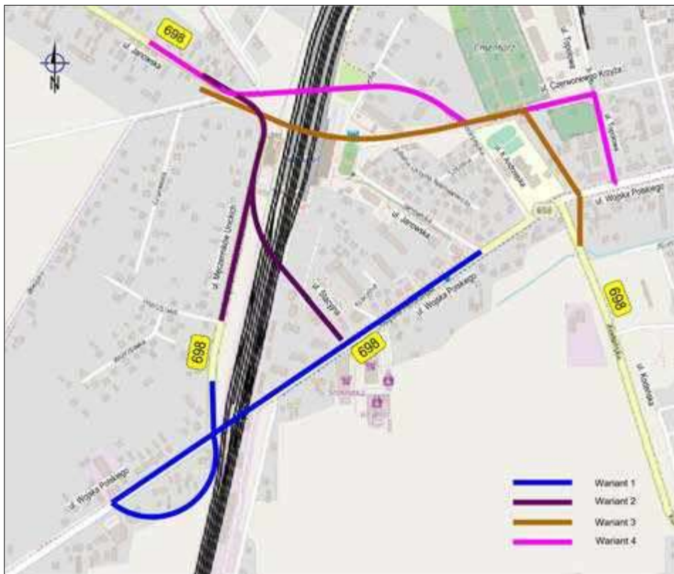
Dotychczas przedstawiono cztery warianty planowanej inwestycji – budowy tunelu lub wiaduktu w Terespole
