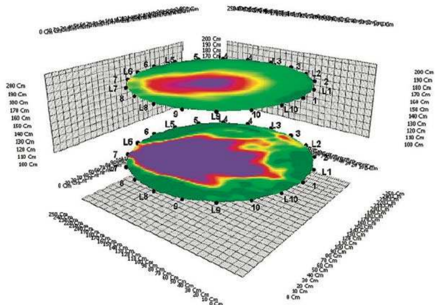
Wynik badania tomografem sonicznym
