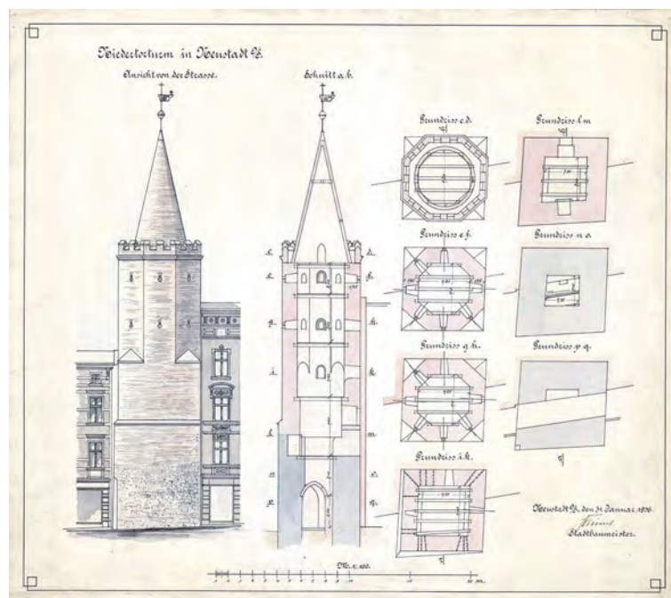
Rysunek inwentaryzacyjny Wieży Bramy Dolnej z 1906 roku
