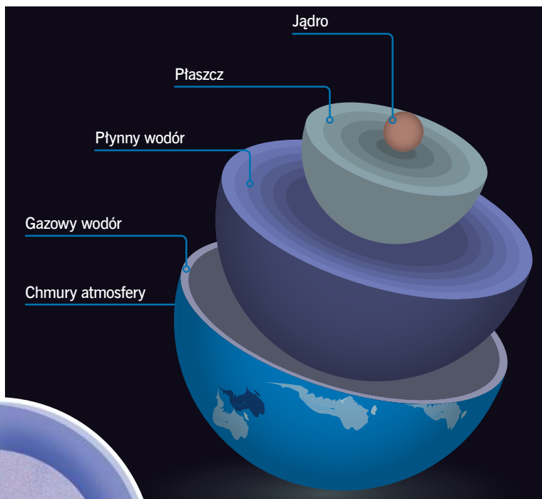
Struktura wewnętrzna Neptuna, czyli ósmej, najdalszej planety Układu Słonecznego
