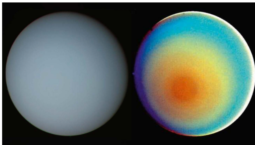
Zdjęcia Urana. Po lewej – barwy prawdziwe. Po prawej – kompilacja obrazów uzyskanych przez sondę Voyager, która przelatywała koło planety w 1986 r.
