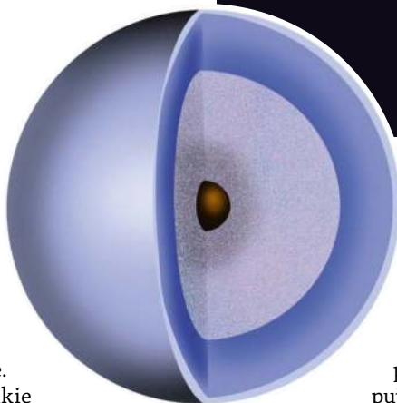
Struktura wewnętrzna Neptuna, czyli ósmej, najdalszej planety Układu Słonecznego
