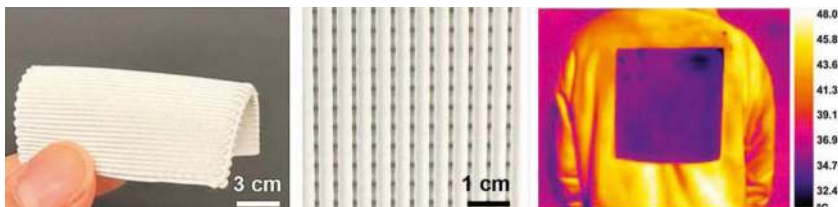
Struktura wielofunkcyjnej tkaniny, która chłodzi lub grzeje.
