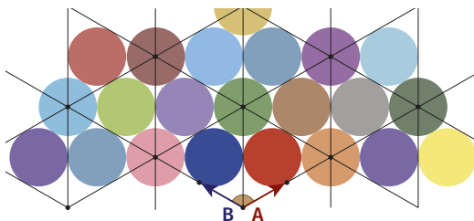
Rysunek 6. Diagram Dynkina A_2 daje wskazówkę, jak najczęściej rozmieszczać koła na płaszczyźnie
