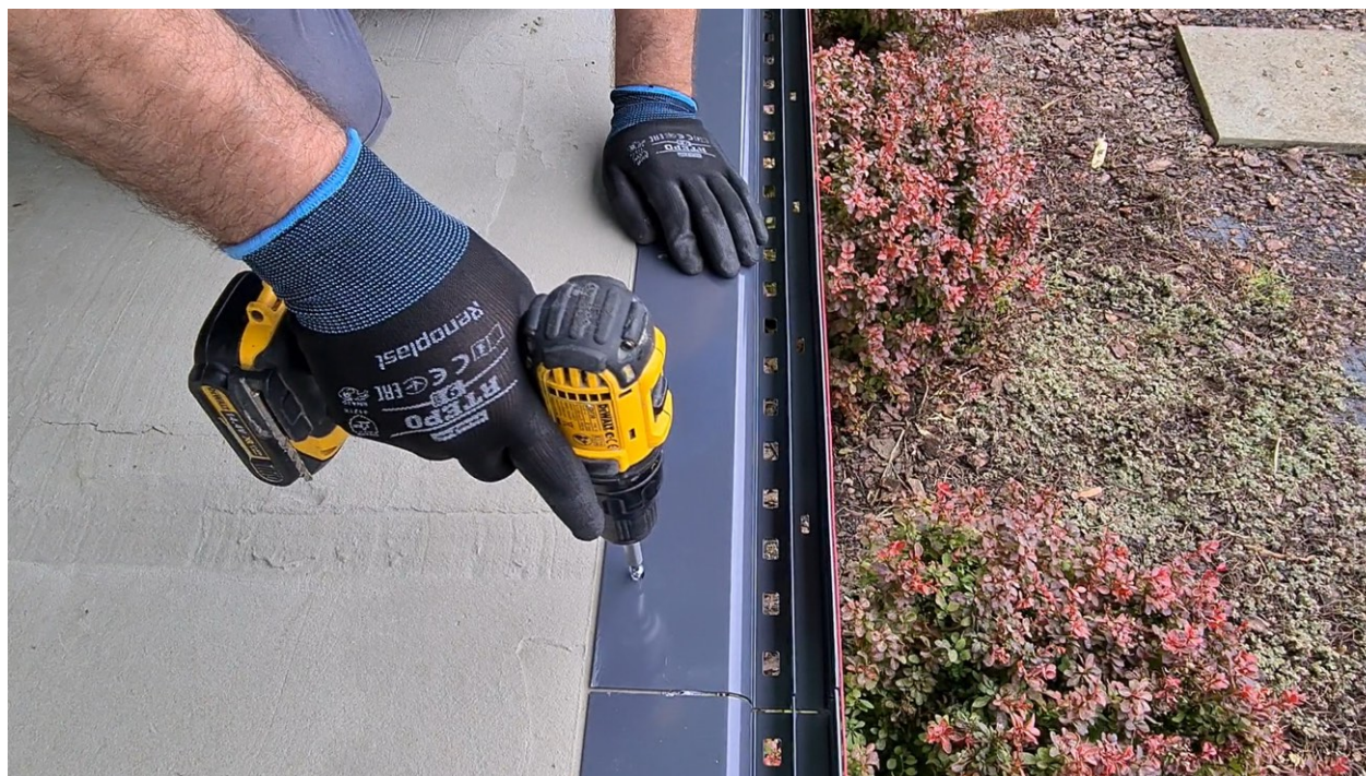
Fot. 2 Montaż profilu okapowego
