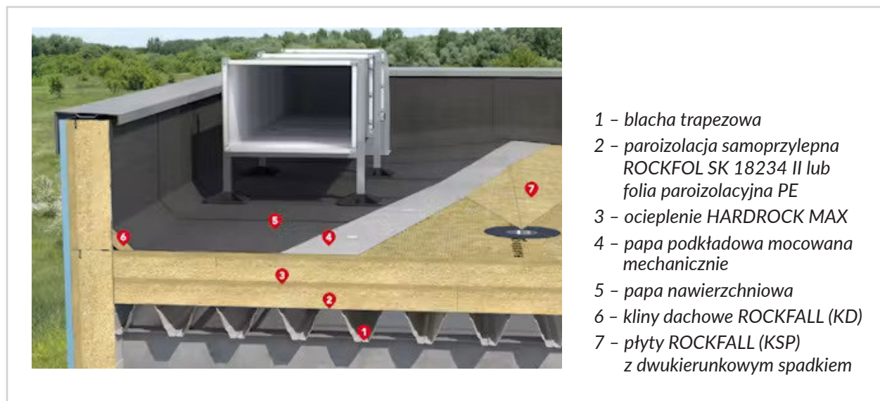
Rys. 1 Schemat ocieplenia dachu płaskiego na blasze trapezowej – warstwy mocowane łącznikami; źródło https://www.rockwool.com/pl , dostęp: maj 2026 r.
