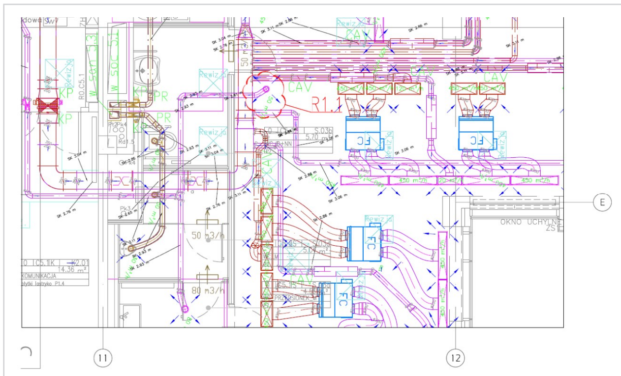
Przykładowy fragment projektu instalacji wentylacji, klimatyzacji i przeciwpożarowej w jednym z budynków AGH; archiwum dokumentów przetargowych AGH
