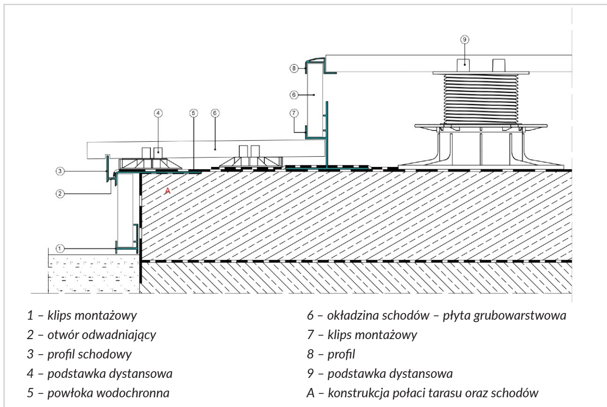
Rys. 2 Przejście taras – schody
