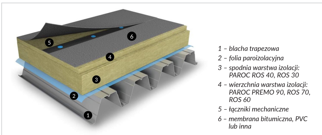
Rys. 2 Izolacja dachu z blachy trapezowej – płyty standardowe; źródło https://www.paroc.com/pl-pl , dostęp: maj 2026 r.
