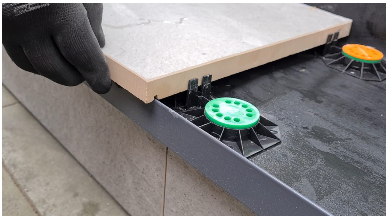
Fot. 9 Podstawka dystansowa i płyta stopnicy
