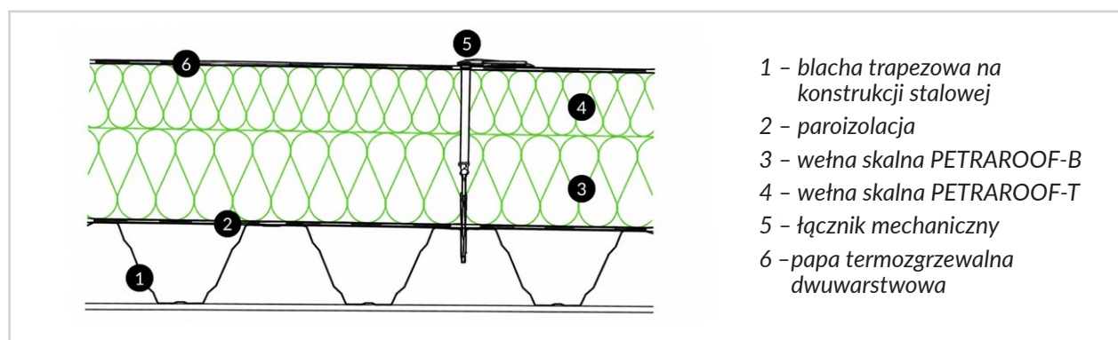
Rys. 4 Izolacja dwuwarstwowa dachu płaskiego na blasze trapezowej; źródło https://www.petalana.eu/pl , dostęp: maj 2026 r.
