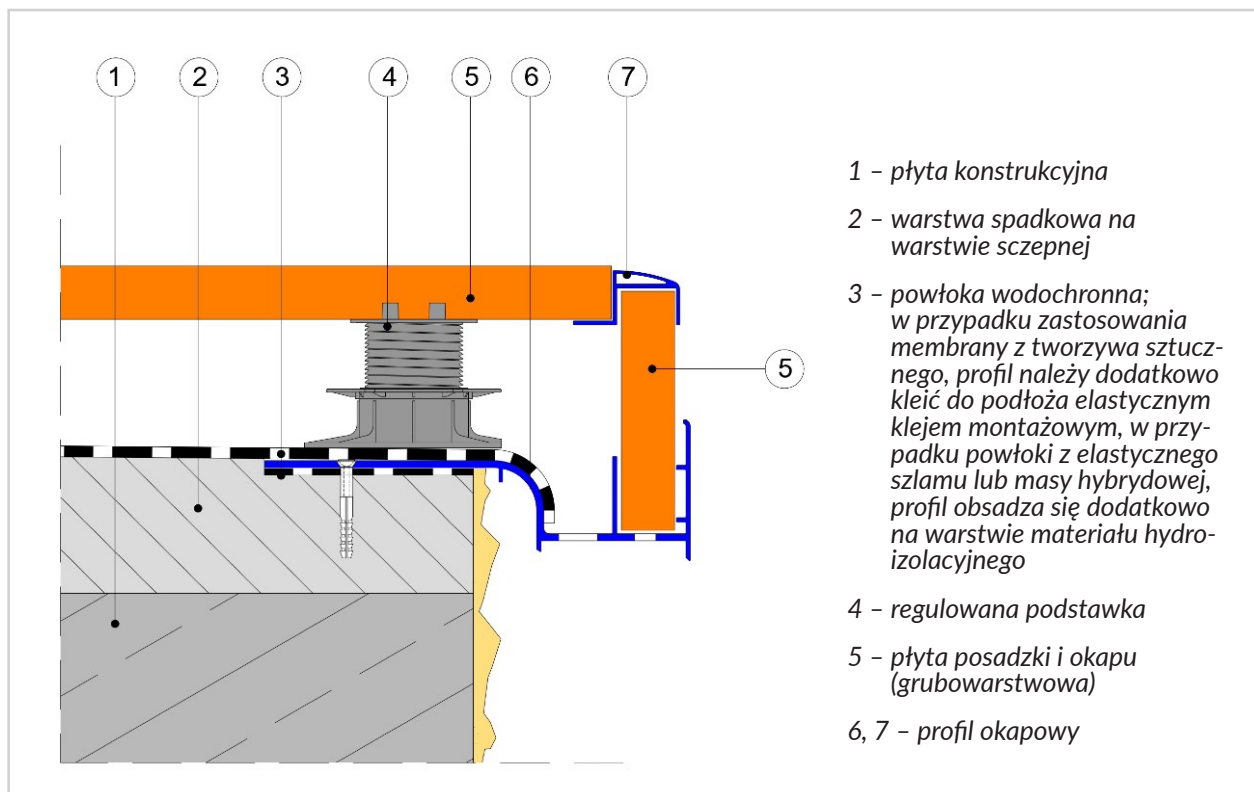
Rys. 1 Budowa warstwy użytkowej tarasu (przekrój połaci) i sposób montażu profilu okapowego
