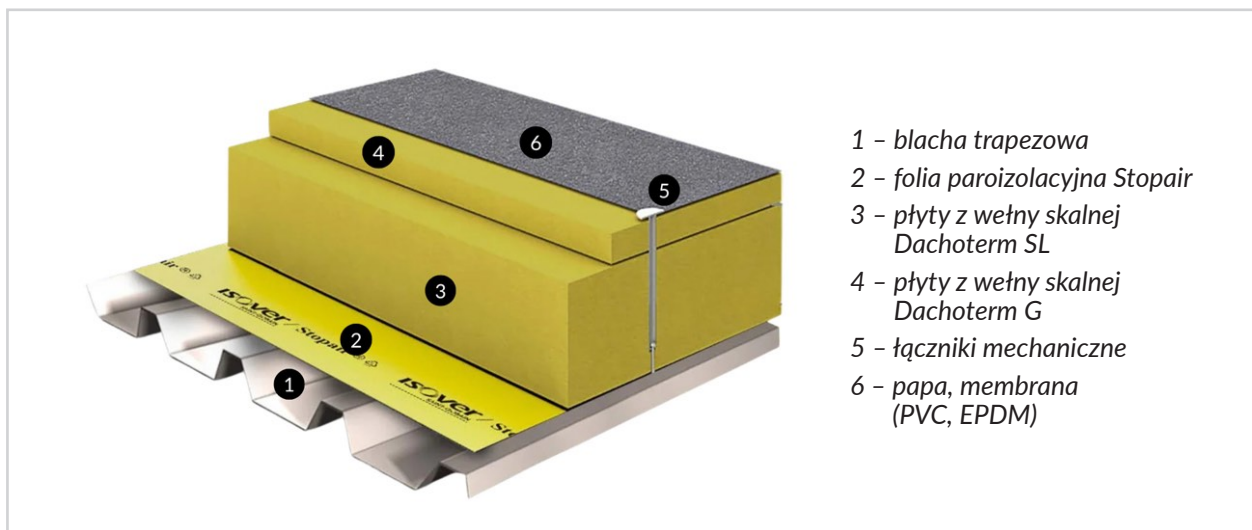
Rys. 3 Ocieplenie dachu z blachy trapezowej – tzw. Srebrny Dach; źródło https://www.isover.pl , dostęp: maj 2026 r.
