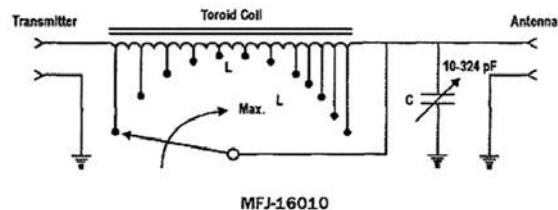
Schemat skrzynki do LW wg MFJ 16010
