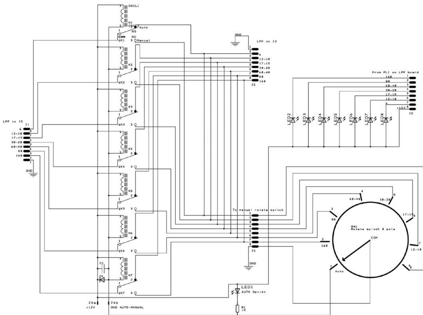
Rys. 3. Schemat układu Auto-manual z przetłącznikiem filtrów LPF
