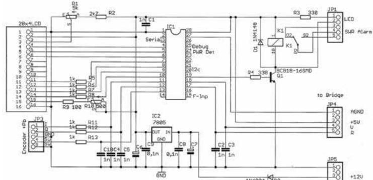
Rys. 2. Schemat układu pomiarowego wg TP3LJ oraz płytka PCB z rozmieszczeniem elementów układu pomiarowego
