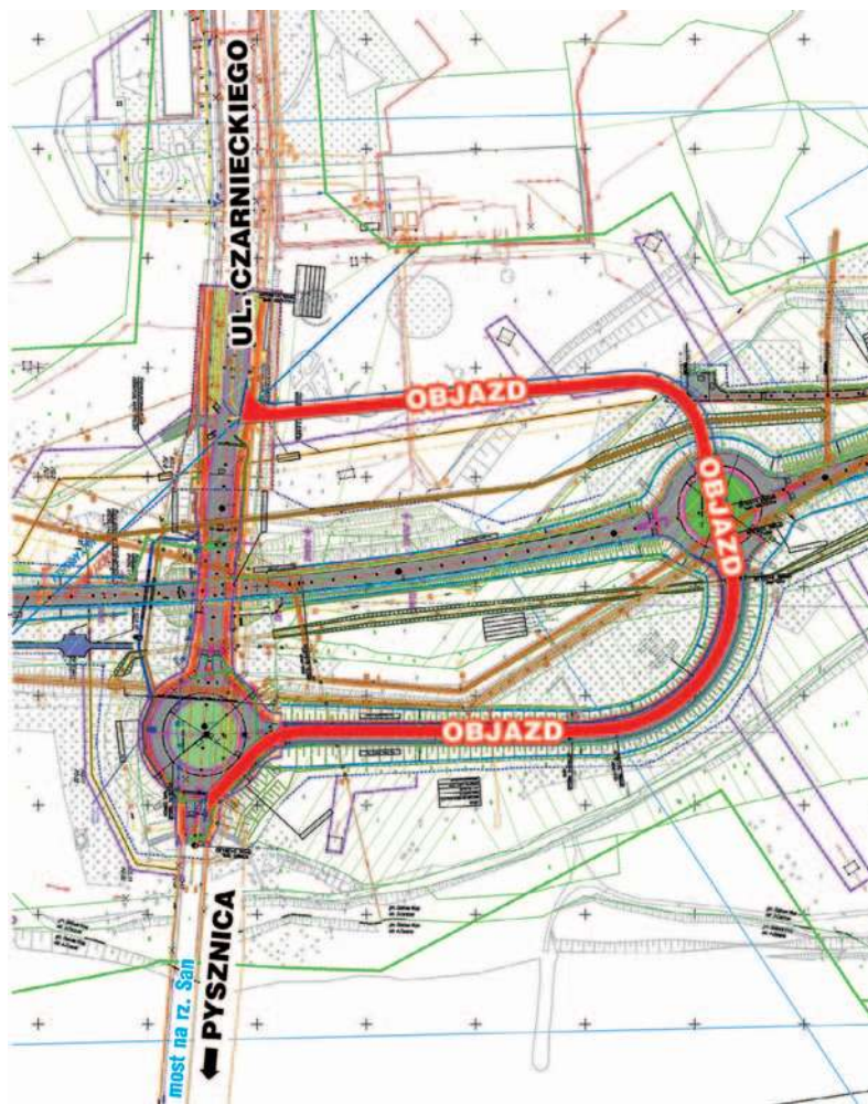
Schemat budowy tymczasowego objazdu, umożliwiającego ruch na drodze powiatowej z Pysznicy do Stalowej Woli
