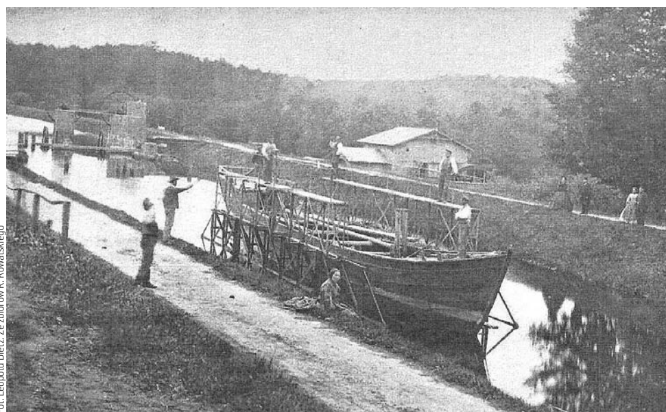
Barka oberlandzka na kratownicowym wózku w Buczyńcu – 1862 r. Widać złożony maszt i jego jarzmo. Z lewej strony zdjęcia - poręcze do wiązania koni
