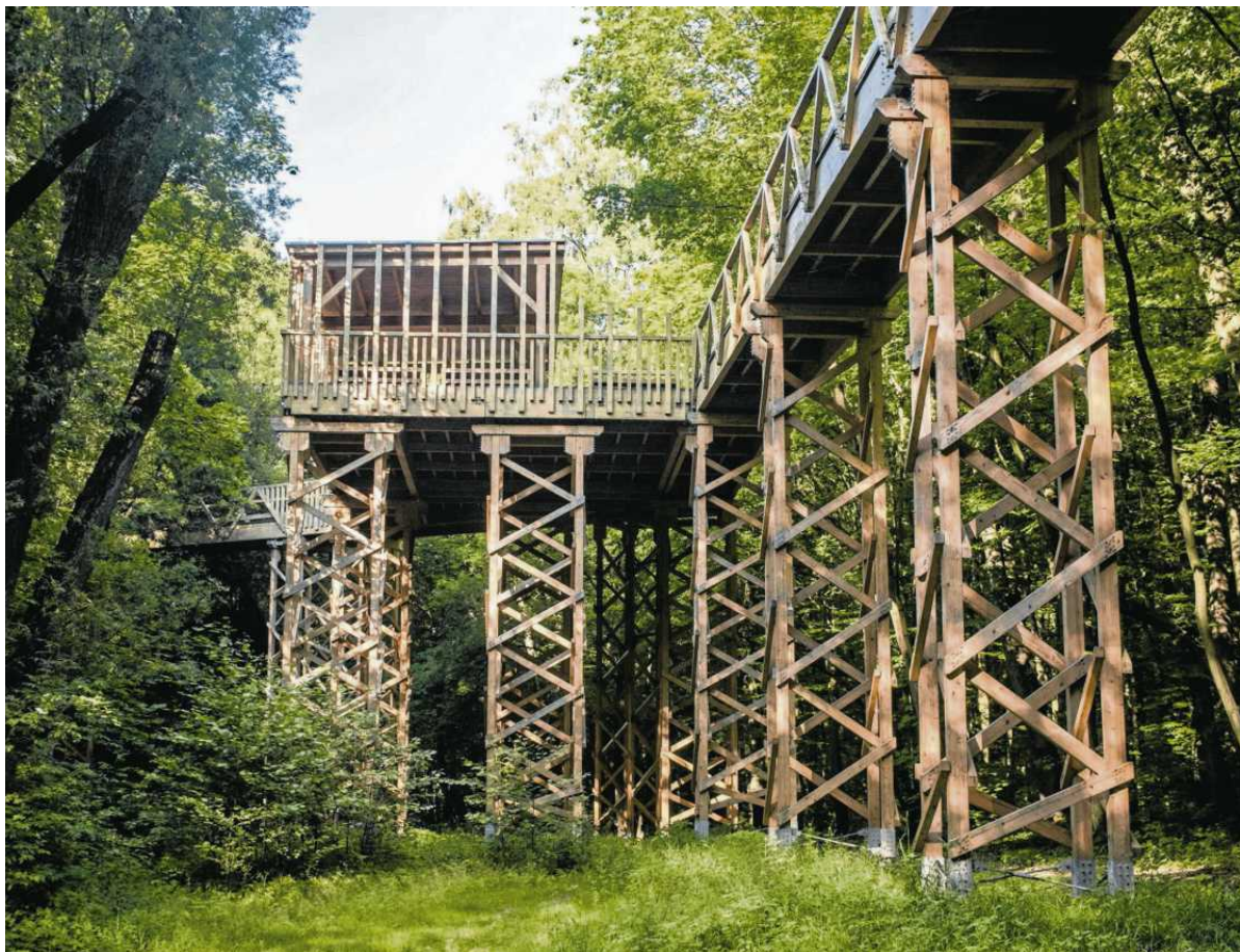
• Kładka pieszo-rowerowa nad rzeką Szklarka FOT. RAFAL POZORSKI / AGENCJA WYBORCZA.PL
