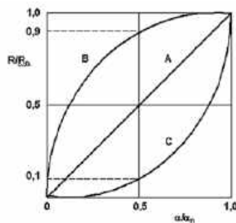
Rys. 2. Oznaczenia charakterystyki potencjometrów polskiej produkcji
