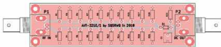
Rys. 5. Rozmieszczenie elementów na płytce drukowanej AVT 3210
