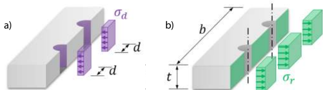
Rys. 4. Naprężenia normalne: a) docisk powierzchniowy trzpienia do blachy, b) rozciąganie blachy w osłabionym otworami przekroju
