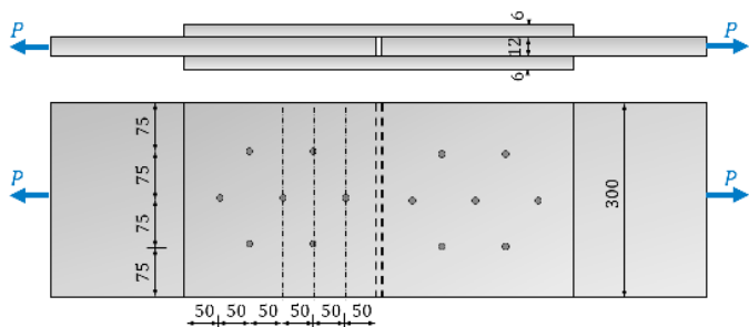
Rys. 6. Przykład obliczeniowy – połączenie nitowane nakładkowe
