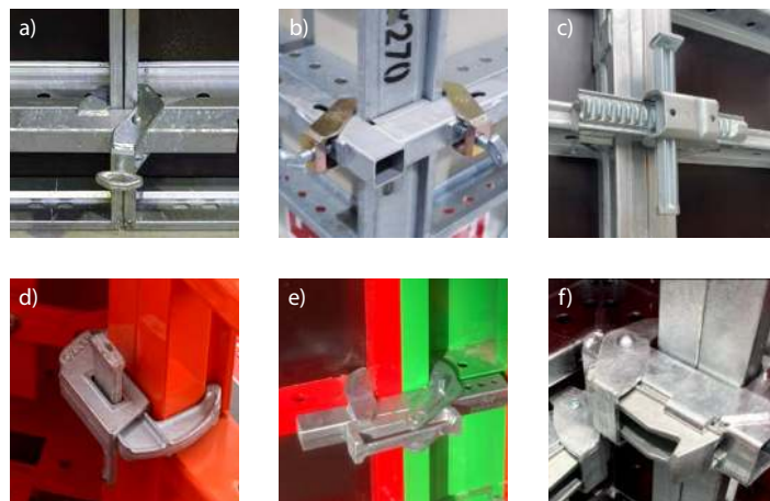
Fot. 2. Przykłady różnych rozwiązań zamków szalunkowych: a) zamek śrubowy, b) zamek śrubowy narożny, c) zamek z pionowym klinem, d) odlany zamek z pionowym klinem, e) i f) zamek z poziomym klinem
