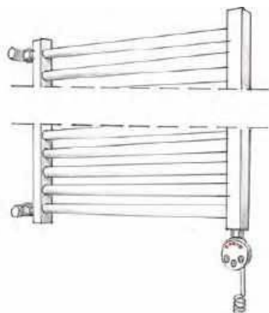
Rys. 4 Podłączenie boczne grzejnika. Grzałkę należy umieścić wówczas po jego przeciwnej stronie.
