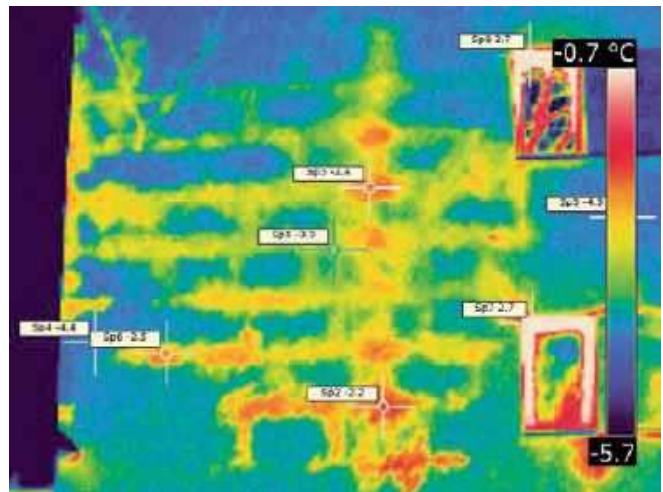
Na zdjęciu wykonanym kamerą termowizyjną widać miejsca, przez które z budynku ucieka ciepło. ENERG-DOM
