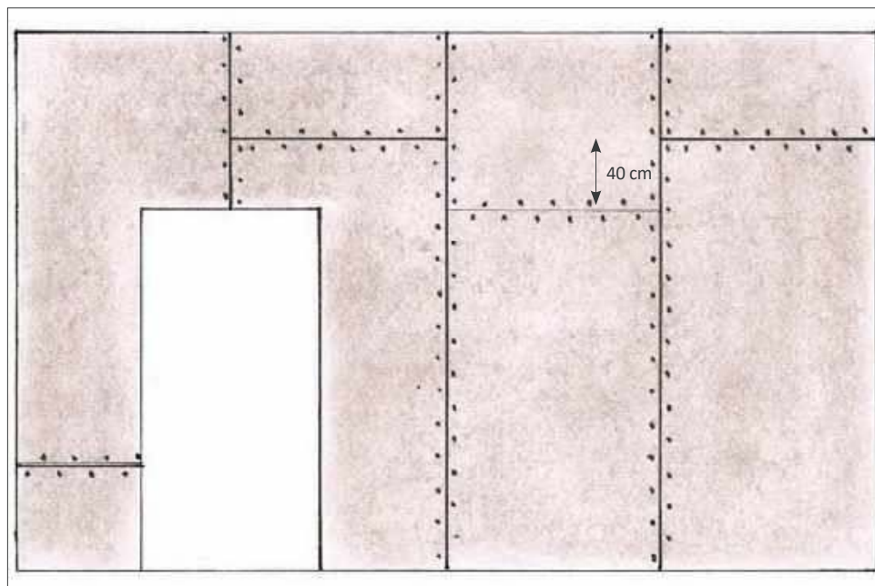
🔧 Poziome łączenia układanych obok siebie karton-gipsów mają być przesunięte o przynajmniej 40 cm. Wokół drzwi płyty wycina się w L.
