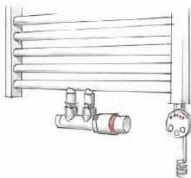
Rys. 2 Podłączenie centralne dolne, tzw. D50. Sprawdźmy po której stronie podłączenie dopuszcza producent.
