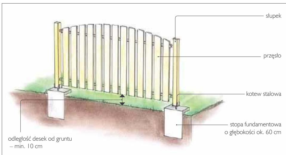
📌 Pod ogrodzenie z lekkich przęseł drewnianych bez podmurówki wystarcza fundament punktowy wykonywany pod słupkami.
