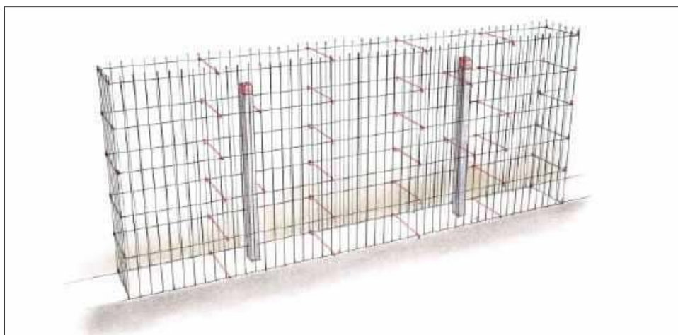
📌 Kosze gabionowe powstają z połączenia panelu przedniego, tylnego i bocznych przy użyciu specjalnych spinek i łączników.
