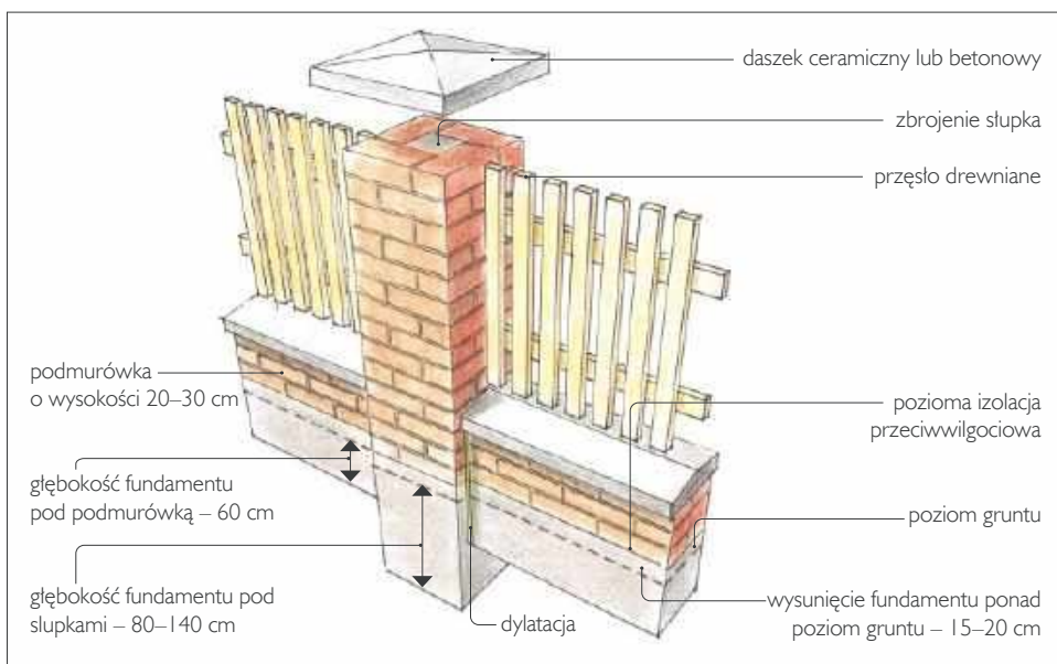
📌 Sposób posadowienia ogrodzenia z murowanym cokołem i słupkami.
