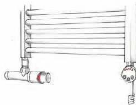
Rys. 3 Podłączenie dolne przez specjalny zawór rurowy. Zasilanie i powrót zajmują dzięki niemu tylko jeden króciec grzejnika.
