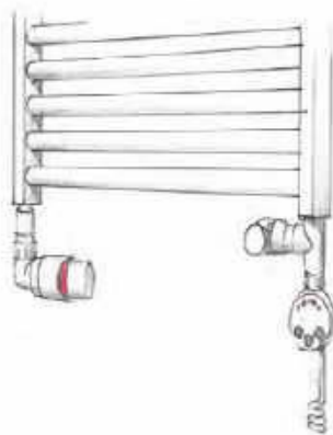
Rys. 1 Klasyczna drabinka o symetrycznym kształcie. Najczęściej grzałkę podłącza się poprzez dodatkowy trójnik założony na powrocie.
