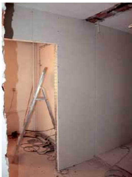
❷ Płyty gipsowo-kartonowe wymagają wykończenia miejsc połączeń poprzez wtopienie taśmy zbrojącej w masę szpachlową. J. WERNER, SINIAT, SINIAT
