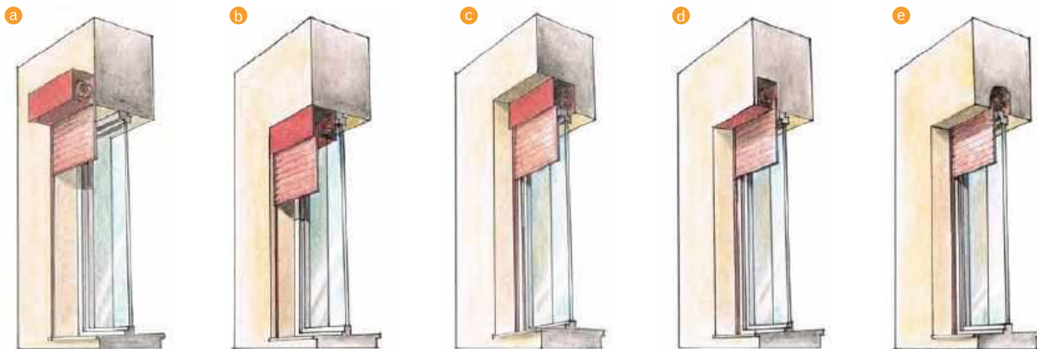
📌 Rodzaje rolet: elewacyjna (a), naokienna prawoskrętnie zwijana (b), nakładana (c), do zabudowy (d), nadprożowa (e).
