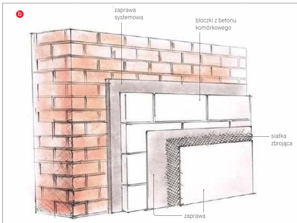
➤ Ściana ocieplona od wewnątrz wełną mineralną (a) i bloczkami z betonu komórkowego (b).
