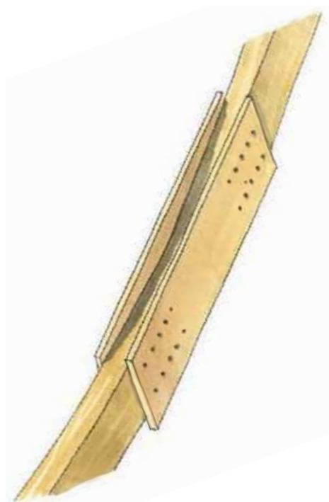
Prosty sposób na wzmocnienie krokwi – nabicie desek z obu stron.
