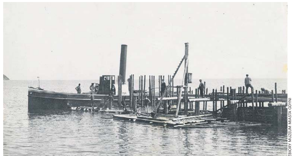
Wbijanie pali pod budowę portu tymczasowego w Gdyni - inż. Tadeusz Wenda na holowniku „Kastor” nadzoruje pracę
