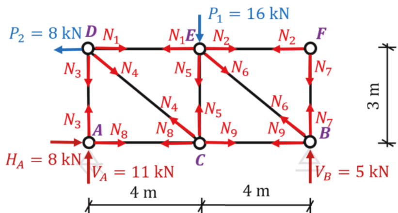
Rys. 9. Schemat sił oddziałujących na węzły kratownicy
