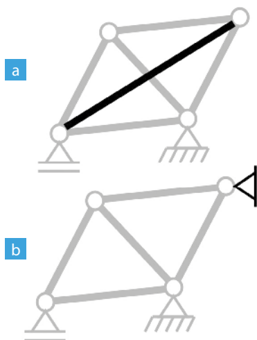
Rys. 5. Przykłady schematów statycznie niewyznaczalnych a) wewnętrznie b) zewnętrznie
