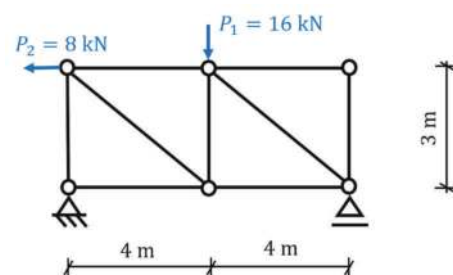
Rys. 6. Schemat statyczny kratownicy
