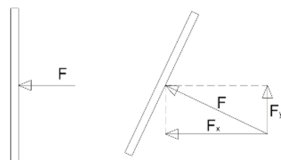
Rys. 1. Siły nacisku na ściany deskowania wywołane parciem mieszanki betonowej; a) deskowanie proste, b) deskowanie nachylone
