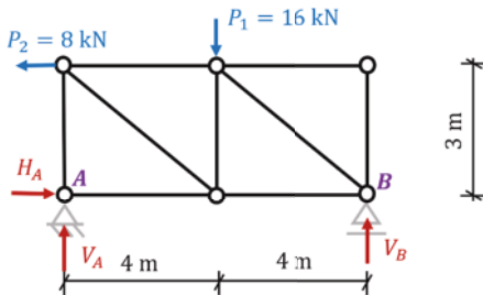
Rys. 7. Schemat obliczeniowy kratownicy osztywnionej z węzłów podporowych
