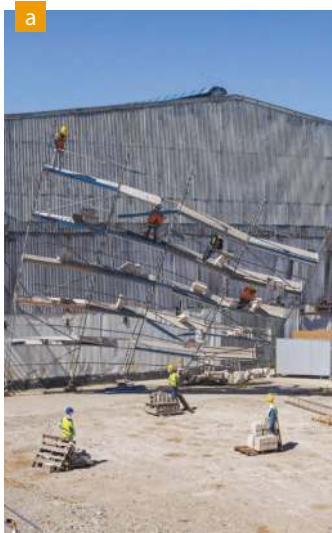
Fot. 6. Kontrolowana katastrofa konstrukcji rusztowania wraz z udzieleniem pierwszej pomocy osobom, które zostały poszkodowane w jej wyniku
