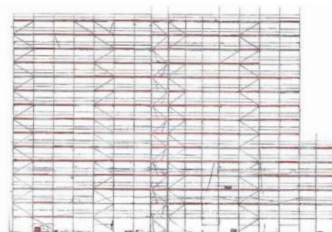
Rys. 6. Widok na fragment zewnętrznej powłoki rusztowania budowlanego – fragment chmury punktów opracowanej za pomocą fotogrametrii [9]
