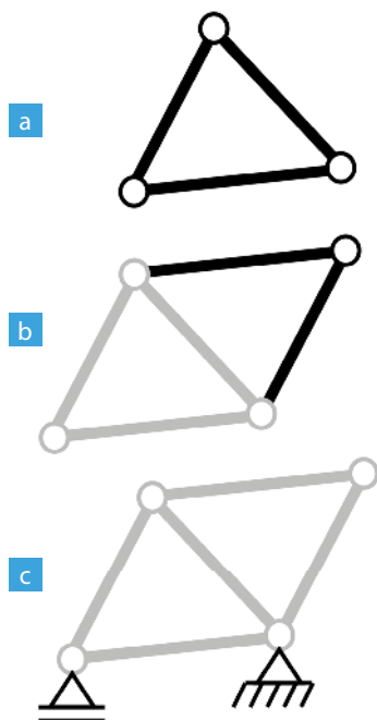
Rys. 4. Konstrukcje prętowe: a) sztywne połączenie trzech prętów ze sobą, b) tworzenie sztywnej kratownicy, c) geometrycznie niezmiennne podparcie kratownicy
