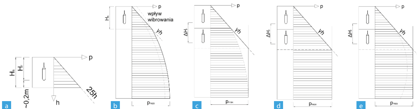
Rys. 2. Rozkład ciśnienia pochodzącego od parcia mieszanki betonowej
