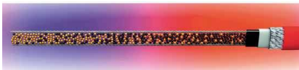
W przewodach samoregulujących pod wpływem zmian temperatury rozluźniają się lub zagęszczają ścieżki przewodzące prąd. Jego przepływowi towarzyszy wydzielanie ciepła. NVENT
