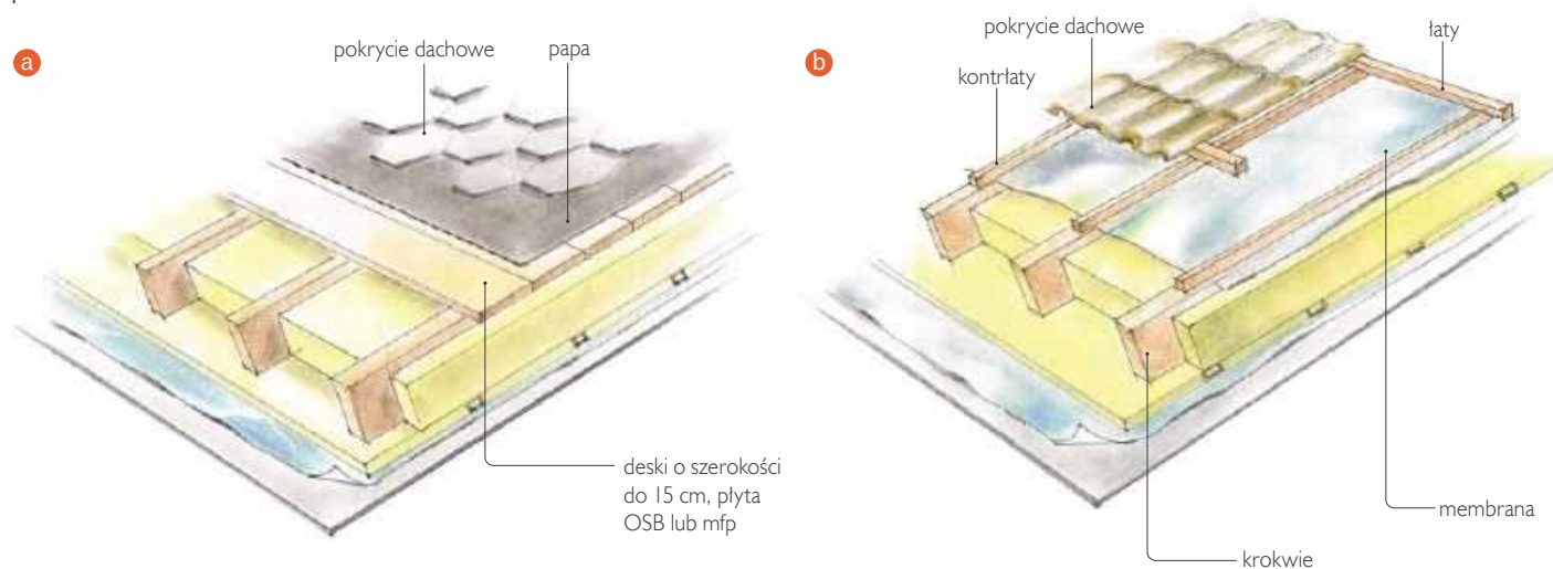
Podkład w formie deskowania (a) oraz rusztu z kontrłąt i łąt (b).
