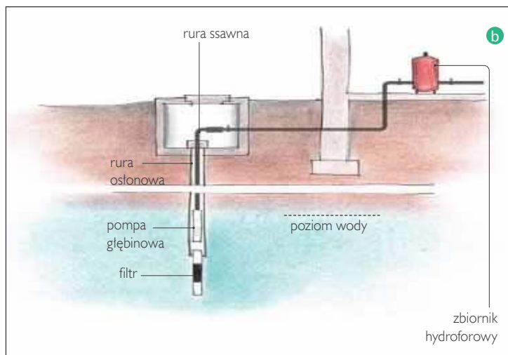
ⓘ Rodzaje studni: wąskorurkowa (b), wiercona (c).
