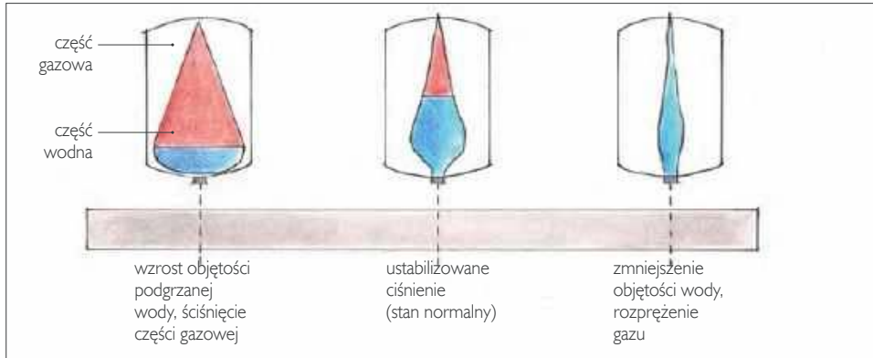
Rys. 1 Wzrost objętości wody po jej podgrzaniu powoduje jej większy napływ do wnętrza naczynia i ściśnięcie części (poduszki) gazowej. W ten sposób ciśnienie wody nie wzrasta ponad miarę.
