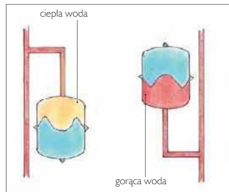
Rys. 4 Założenie naczynia wzbiorczego króćcem przyłączeniowym ku górze zabezpiecza je przed napływem najbardziej gorącej wody.
