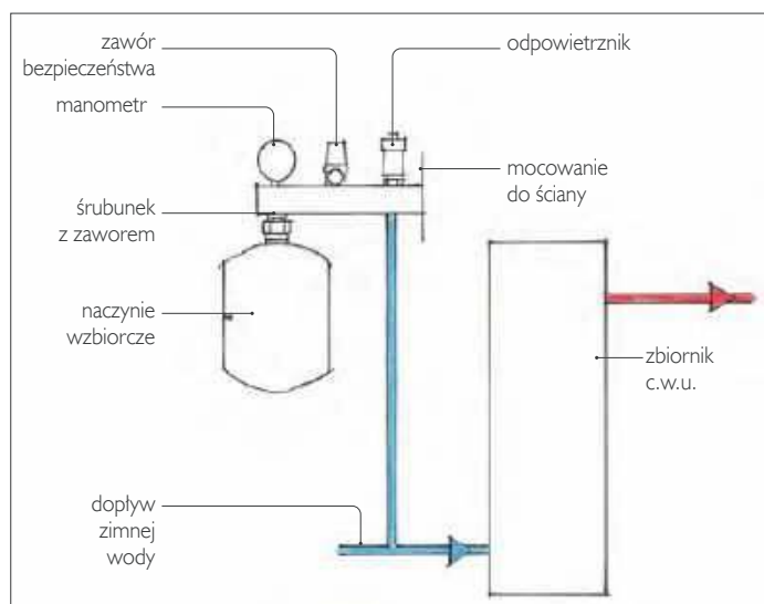
Rys. 3 Grupa bezpieczeństwa to manometr, zawór bezpieczeństwa, odpowietrznik i złączka do naczynia wzbiorczego zamontowane na wspólnej belce przyłączeniowej.
