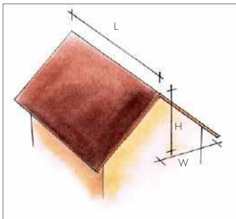
📍 Jeśli nachylenie połaci nie przekracza 10°, przyjmuje się, że EPD jest taka sama jak powierzchnia dachu. Do obliczenia orynnowania bardziej stromych dachów korzysta się ze wzoru, którego symbole wyjaśniono na rysunku: EPD = (W + \frac{1}{2}H) \cdot L
