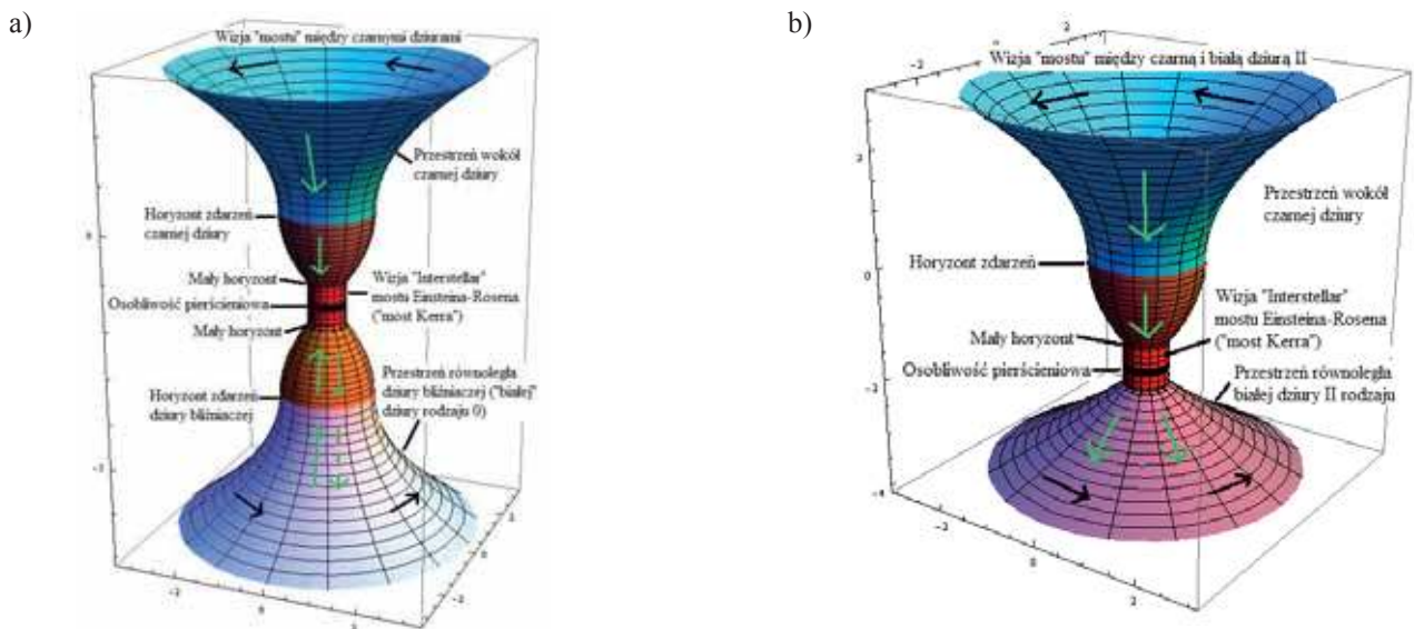
Rys. 5. Wizja „mostu Kerra” przebiegającego około łagodnej osiowości (pierścieniowej) pomiędzy sprzężonymi rotującymi dziurami dla: a) dwóch bliźniaczych czarnych dziur – czyli czarnej dziury i „białej” dziury rodzaju 0; b) czarnej dziury i białej dziury II rodzaju. Wizja jest inspirowana postacią pokładowego astrofizyka Romilly’ego granego przez Davida Gyasi w filmie Interstellar i nawiązuje do rozwiązania Kerra z 1963 r. [12]. W przeciwieństwie do pozostałych rysunków artykułu wizja ta nie ma ścisłego charakteru matematycznego.
