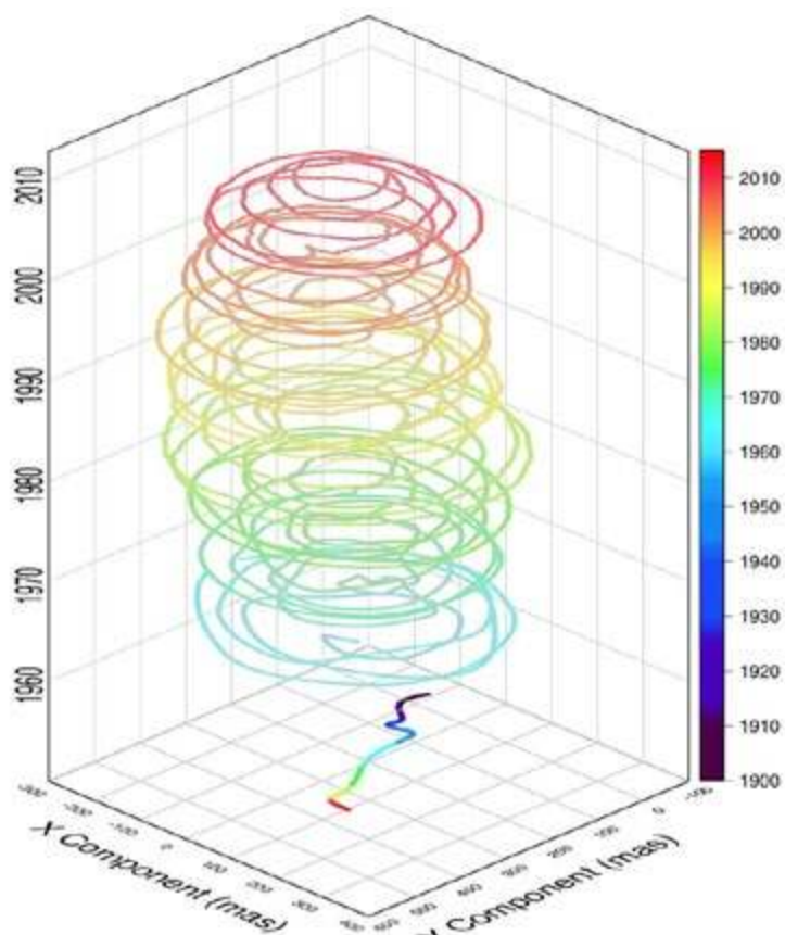
Spirala poloidy z lat 1900-2010, źródło: E.C. Pavlis et al. Use of LARES satellite data for Earth science, 2015.
