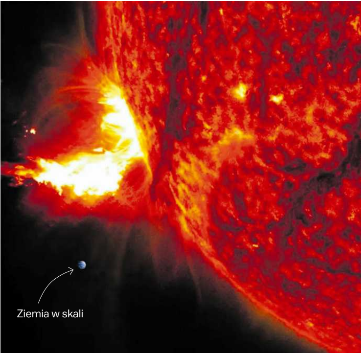
• Rozbłysk słoneczny sfotografowany 27 maja 2024 r. przez obserwatorium słoneczne NASA. Dla porównania – na zdjęciu pokazany jest rozmiar Ziemi FOT. NASA/ SDO
