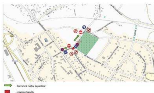
Organizacja ruchu w Dniu Wszystkich Świętych (rejon cmentarzy)
