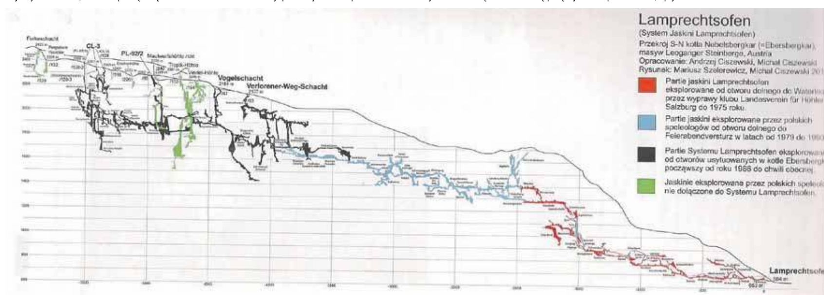
Przekrój Systemu Lamprechtsofen. "Jaskinie" 92/2018
