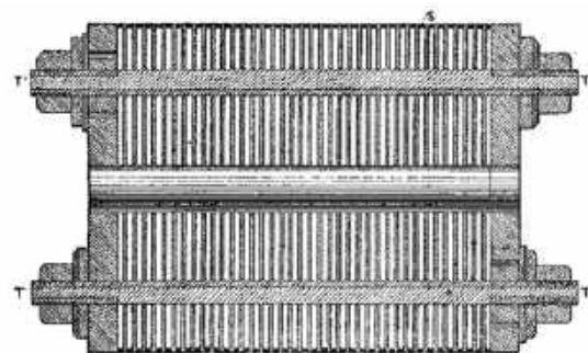
Rys. 6. Walcowy element światłoczuły. T i T' są prętami kontaktowymi, tarcze mosiężne są zakreskowane ukośnie, białe pola pomiędzy nimi to izolacyjne tarcze mikowe, czarna warstwa S to światłoczuła warstwa selenowa pomiędzy dyskami przewodzącymi (źródło: „La Nature”)
