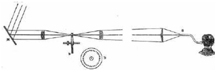
Rys. 9. Telefon muzyczny z tarczą dziurkowaną. Tarcza mogła znaleźć również zastosowanie w transmisji telegraficznej (źródło: „La Revue Scientifique”)
