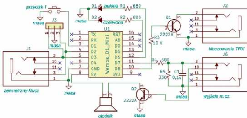
Rys. 1. Schemat ideowy CW Hotline. Gniazdko J2 służy do kluczowania nadajnika za pośrednictwem tranzystora wykonawczego Q1, J1 jest wejściem dla dowolnego zewnętrznego klucza, połączonych równolegle z ewentualnie wbudowanym J3, a J6 jest przeznaczone dla zewnętrznego aktywnego głośnika. Jego podłączenie powoduje wyłączenie głośnika wewnętrznego
