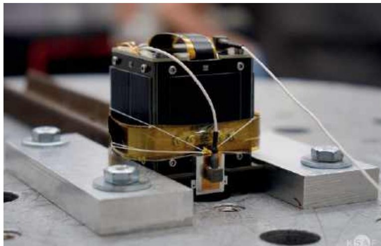
Satelita HYPE podczas testów wibracyjnych przed lotem, fot. KSAF Jakub Kopeć
