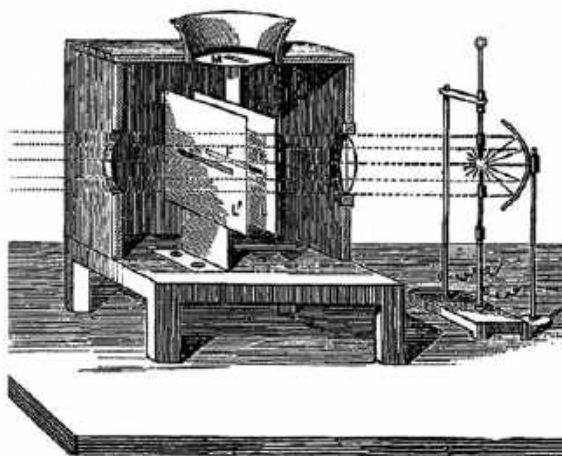
Rys. 4. Modulator jasności zawierający dwie płytki: L (połączoną z membraną M) L' (nieruchomą) mające pojedyncze szczeliny F i F'. Jako źródło światła służy lampa łukowa znajdująca się w ognisku reflektora parabolicznego (źródło: „La Revue Scientifique”)
