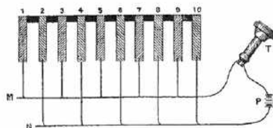
Rys. 7. Zasada naprzemiennego połączenia dysków w obwodzie elektrycznym (źródło: „La Nature”)
