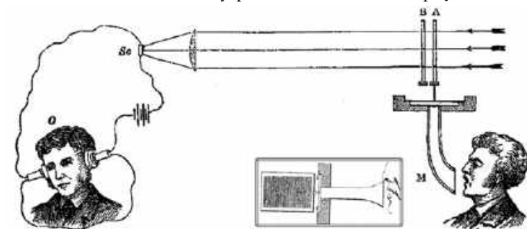
Rys. 3. Modulator szczelinowy składa się z dwóch płytek z wyciętymi szczelinami. Płytką A jest połączona z membraną i porusza się w takt głosu. Płytką B jest nieruchoma. Zmodulowana wiązka światła pada w odbiorniku na selenowy element światłoczuły. W ramce widok płytki od frontu (źródło: „La Nature”, ramka – autor)
