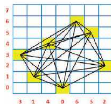
Rys. 4. U góry macierz Costasa dla FT8 zawierająca wartości 3, 1, 4, 0, 6, 5 i 2. Na dolnej ilustracji dowód, że jest to rzeczywiście macierz Costasa
